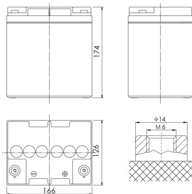
Рисунок 8 - Габаритные размеры аккумулятора
