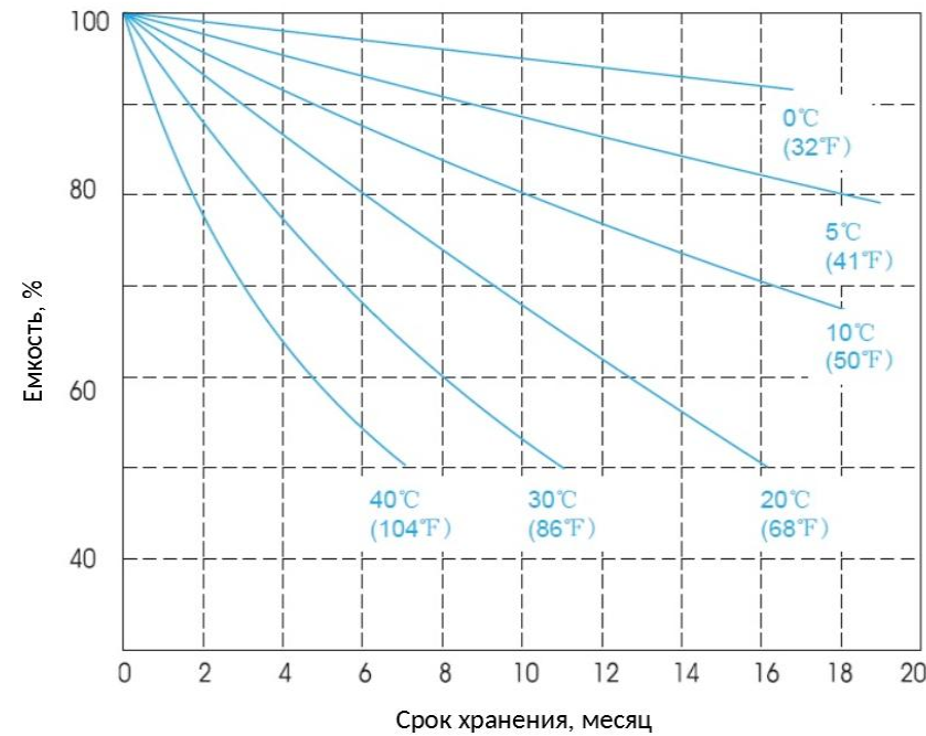
Рисунок 4 - График зависимости остаточной ёмкости аккумулятора от времени хранения при различных температурах окружающей среды
