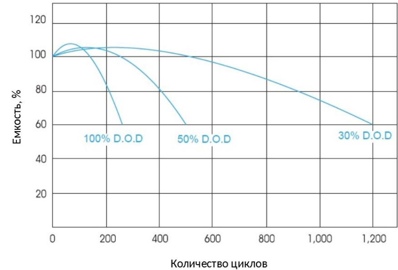
Рисунок 3 - График зависимости ёмкости аккумулятора от количества циклов заряда-разряда при различных глубинах разряда
