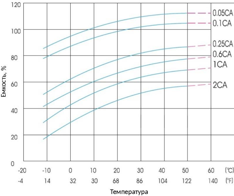
Рисунок 5 - График снижения ёмкости в зависимости от температуры
