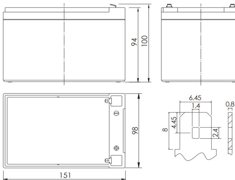
Рисунок 8 - Габаритные размеры аккумулятора
