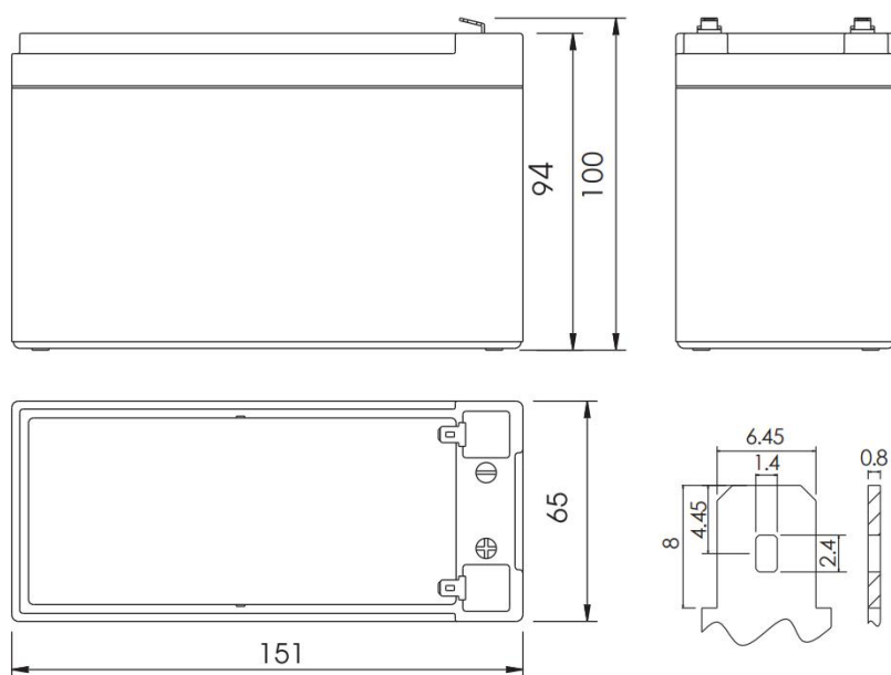
Рисунок 8 - Габаритные размеры аккумулятора
