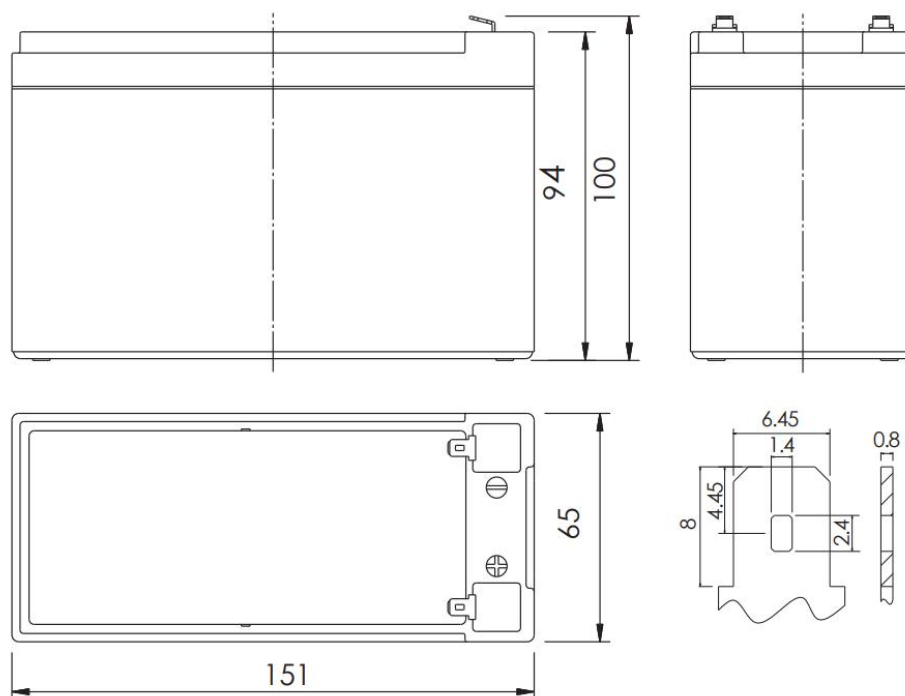
Рисунок 8 - Габаритные размеры аккумулятора
