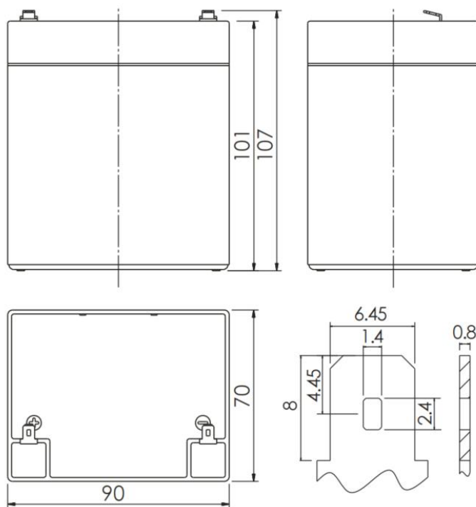
Рисунок 8 - Габаритные размеры аккумулятора
