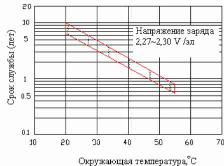
Зависимость срока службы от окружающей температуры
