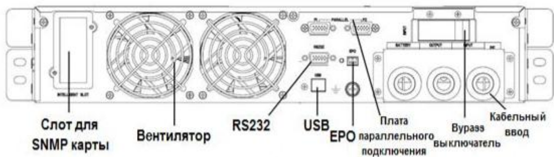
Рисунок 2 - Задняя панель ИБП
