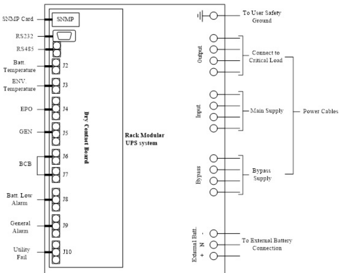
Рисунок 20 Схема подключения
