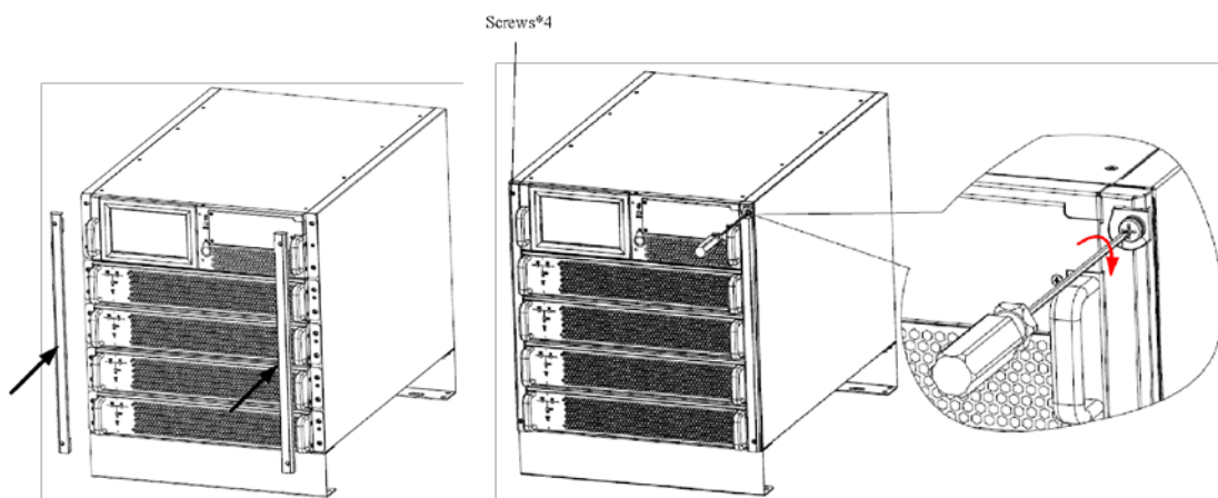
(а) Снятие декоративных планок (б) Установка силового модуля
