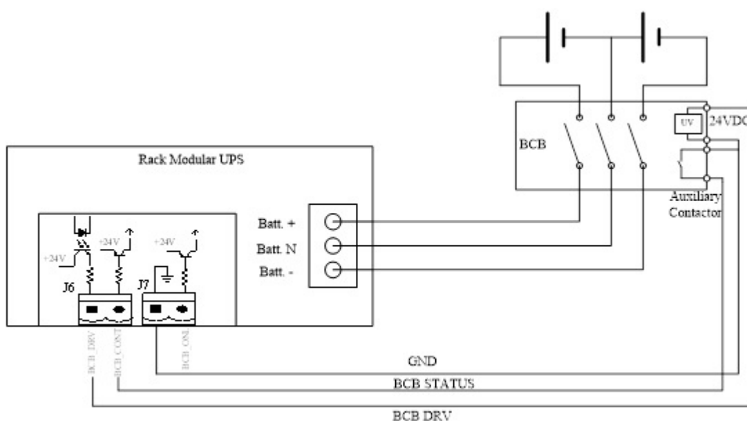
Рисунок 21 Схема подключения внешних АКБ
