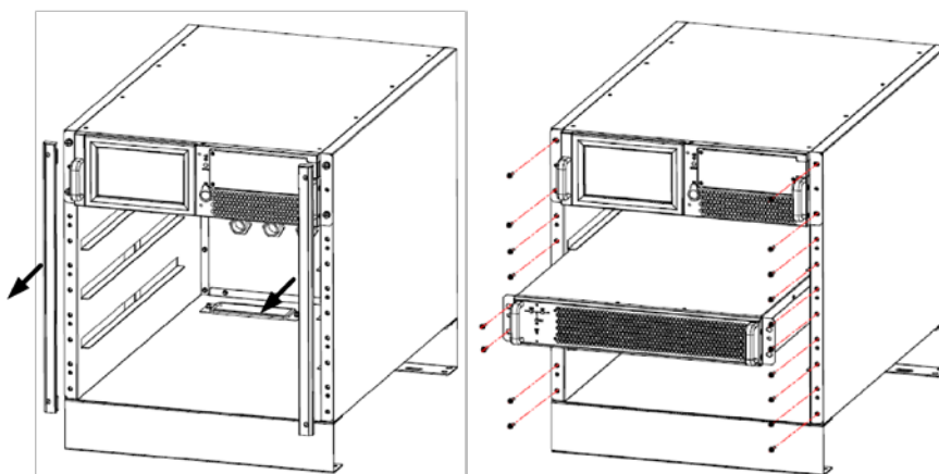
(а) Снятие декоративных планок (б) Установка силового модуля
