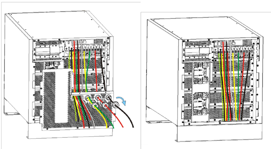
(а) Кабельный ввод в 2х и 4х модульном шасси
