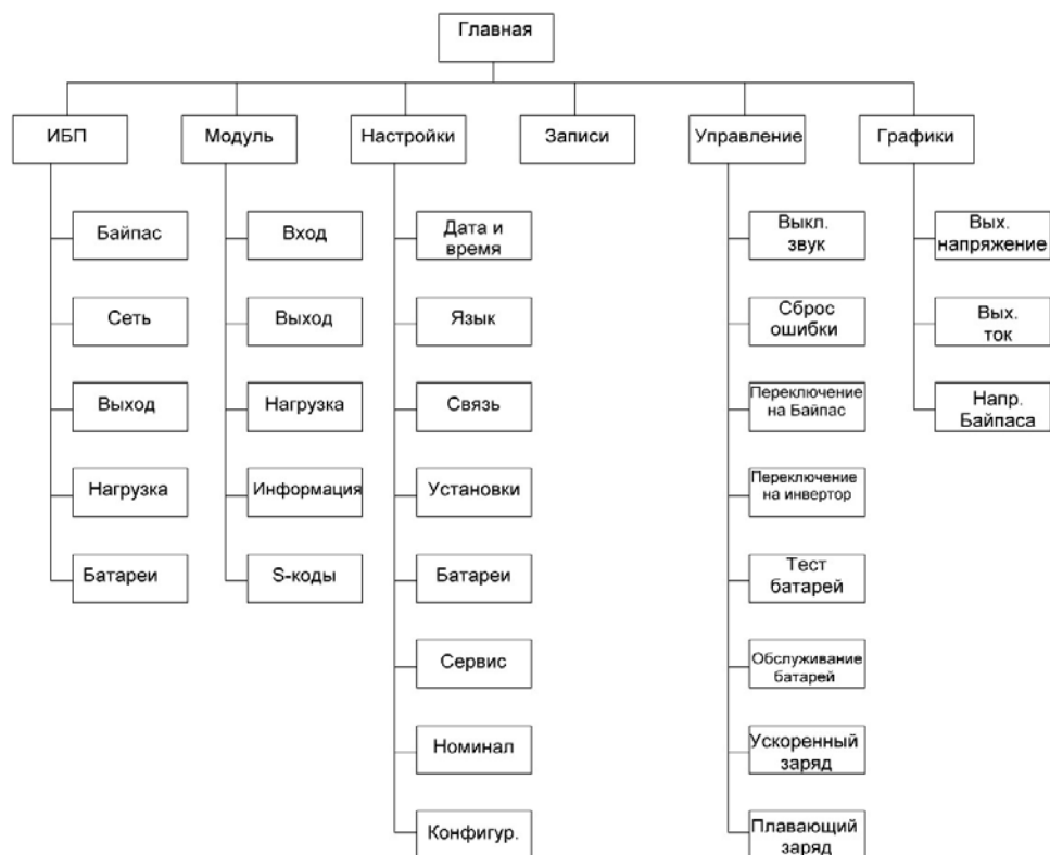
Рис. 7-3: Структура меню
