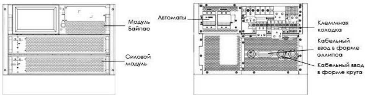
Рисунок 4 – Шасси ИБП с 2 силовыми модулями
