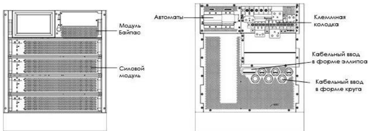
Рисунок 2 – Шасси ИБП с 4 силовыми модулями
