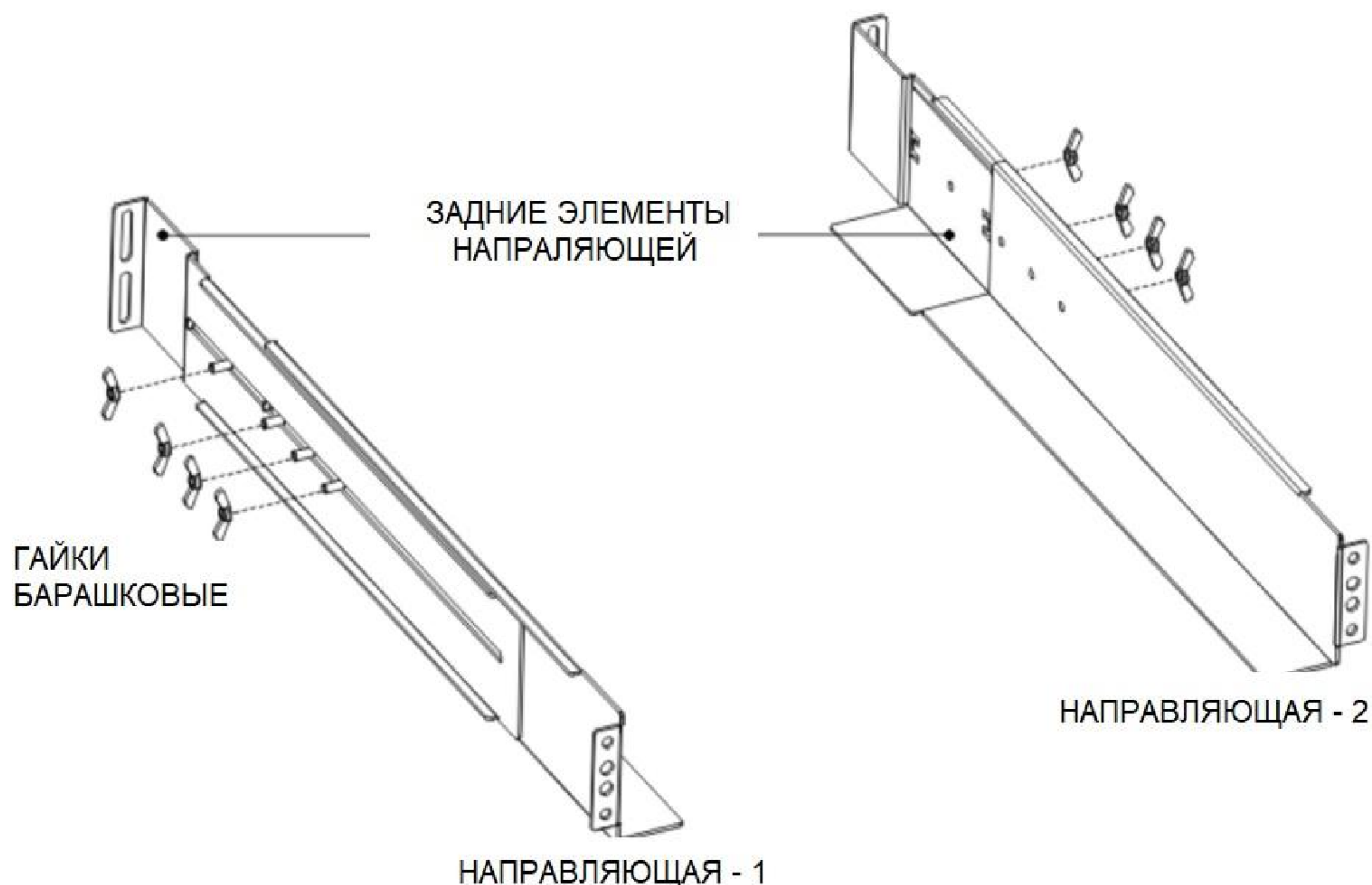
Рис.5 — Сборка направляющих
