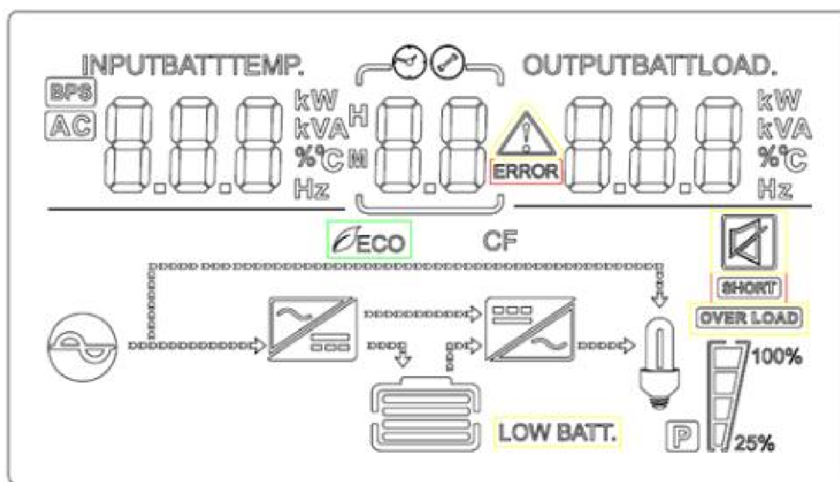
Рис. 18 — ЖК-дисплей
