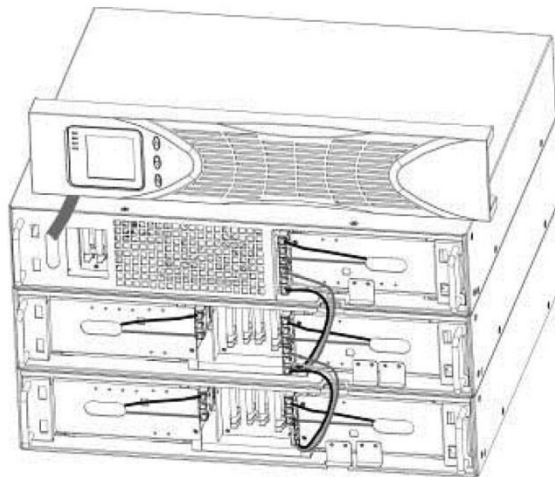
Рисунок 14 – Подключение ЕВР
