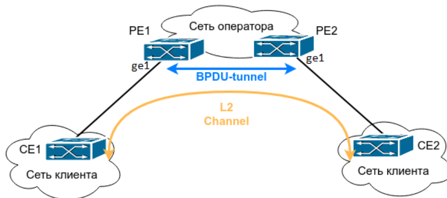
Рис. 8: BPDU-Tunnel
