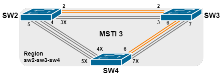
Рис. 13: Топология MSTI 3
