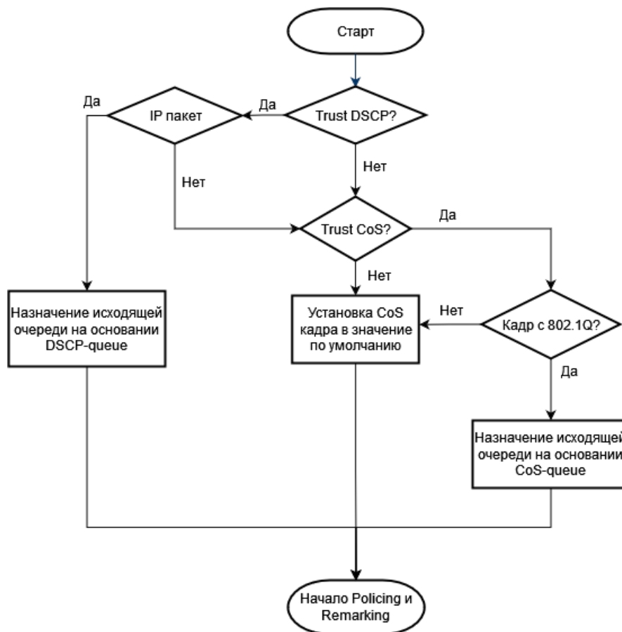
Рис. 18: Процесс классификации пакетов
