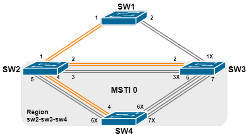
Рис. 12: Топология MSTI 0
