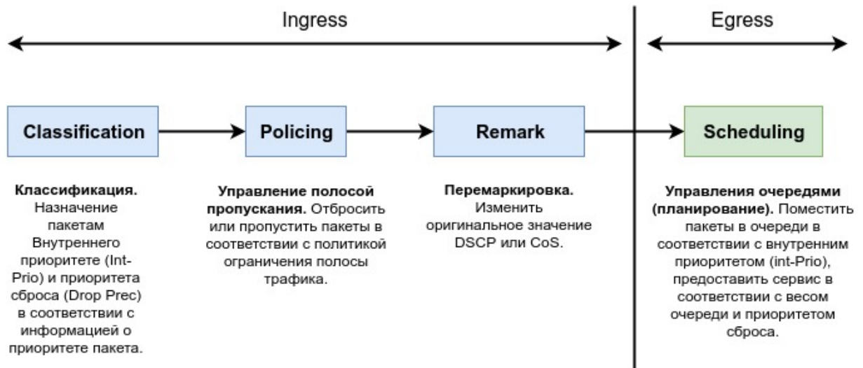
Рис. 17: Базовая модель QoS
