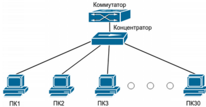
Рис. 29: Конфигурация АМ
