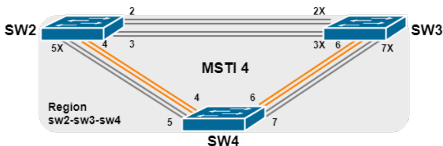
Рис. 14: Топология MSTI 4
