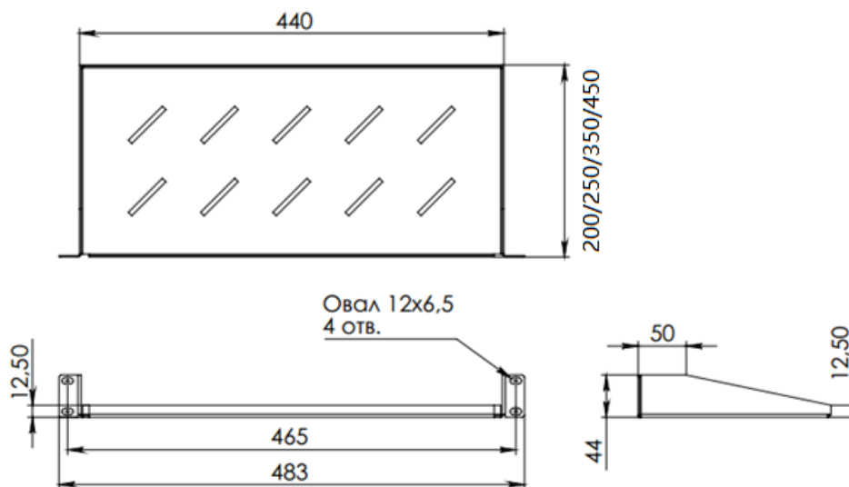
РИСУНОК 2 – ГАБАРИТНЫЕ РАЗМЕРЫ
