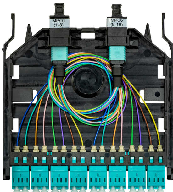
Рисунок 2 - Внутренний конструктив
