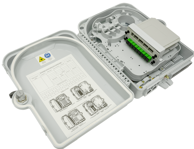
Рисунок 2 - Внутренний конструктив
