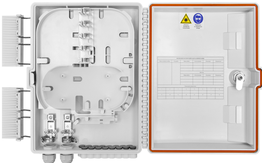
Рисунок 2 - Внутренний конструктив
