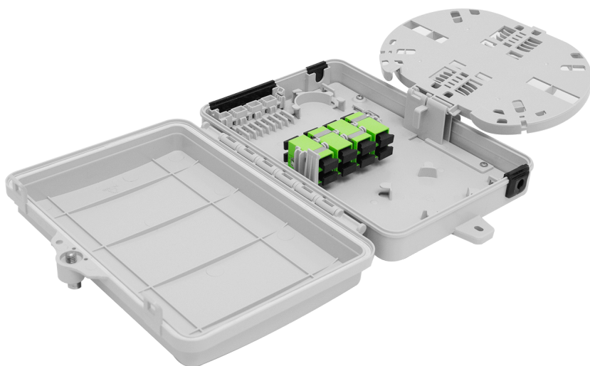
Рисунок 2 - Внутренний конструктив
