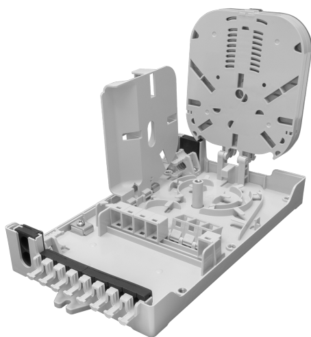
Рисунок 2 - Внутренний конструктив
