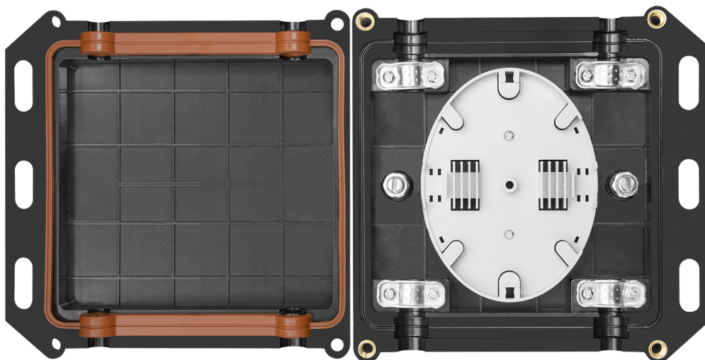
Рисунок 2 - Внутренний конструктив
