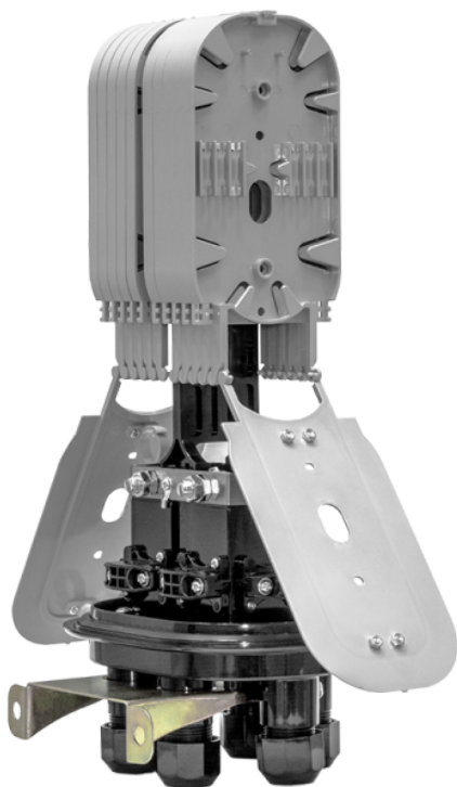
Рисунок 2 - Внутренний конструктив
