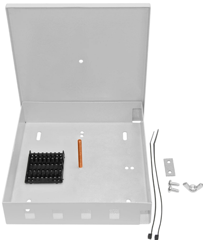
Рисунок 2 - Внутренний конструктив
