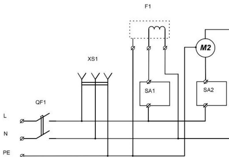
Рисунок 8 - Схема электрическая принципиальная
