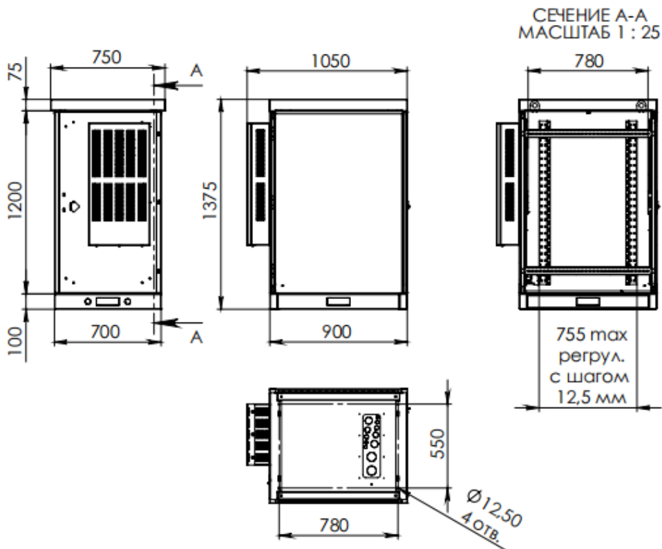
РИСУНОК 3 – ГАБАРИТЫ И РАЗМЕРЫ
