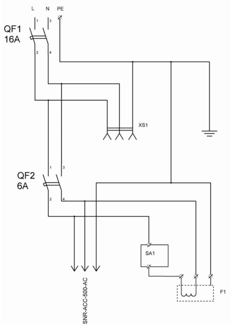
РИСУНОК 4 – СХЕМА ЭЛЕКТРИЧЕСКАЯ ПРИНЦИПАЛЬНАЯ
