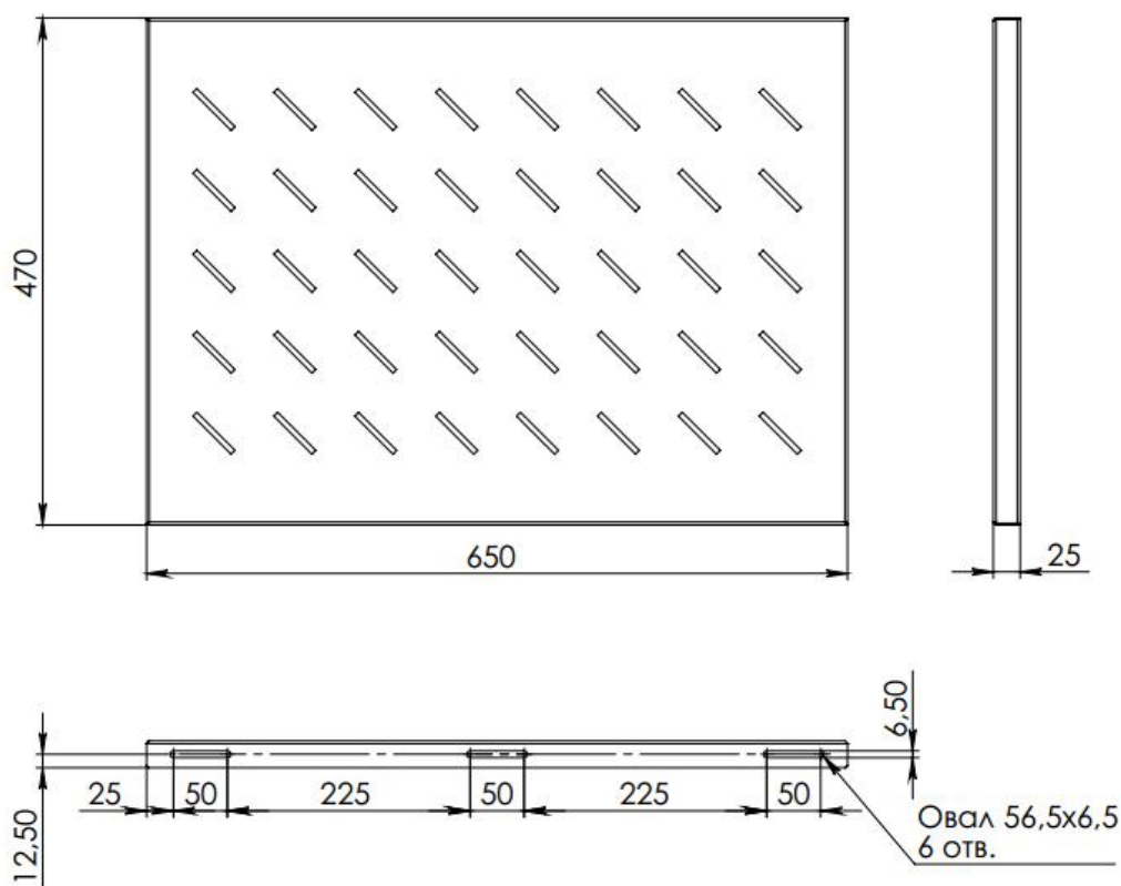
Рисунок 2 - Габаритные размеры
