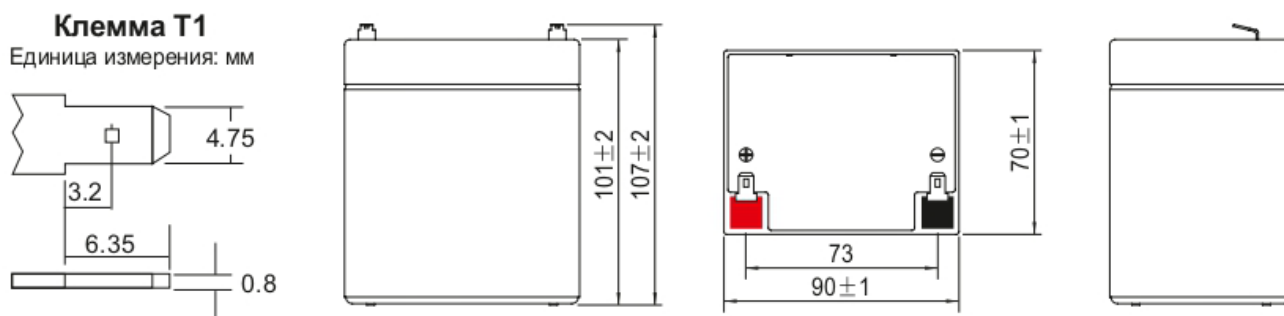
Рисунок 8 – Габаритные размеры аккумулятора
