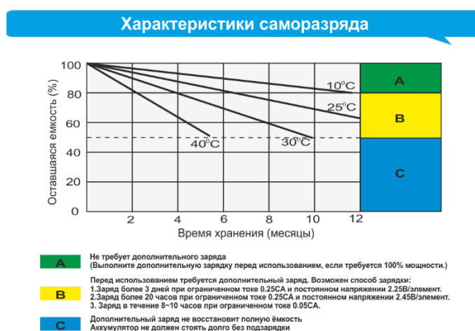
Рисунок 6 – Характеристики саморазряда
