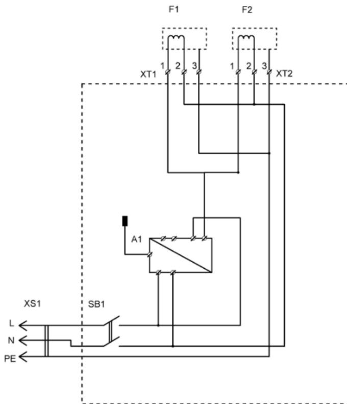
РИСУНОК 4 – СХЕМА ЭЛЕКТРИЧЕСКАЯ ПРИНЦИПИАЛЬНАЯ
