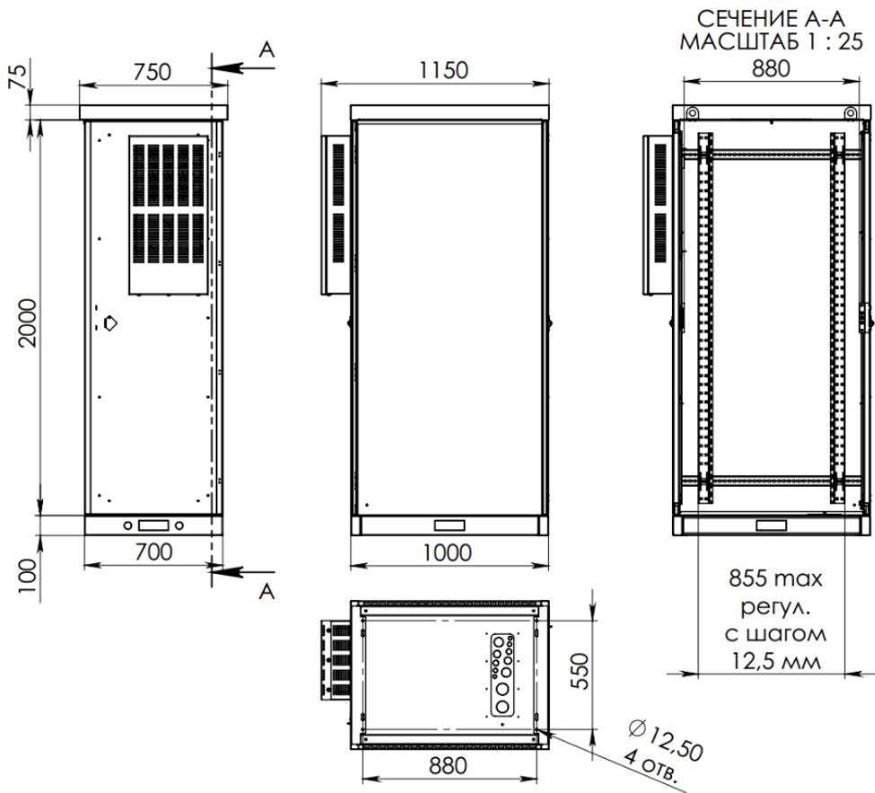
РИСУНОК 3 – ГАБАРИТЫ И РАЗМЕРЫ
