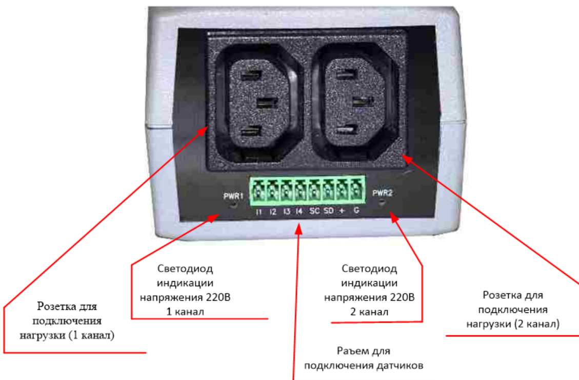
Рисунок 5 – Задняя панель (устройства NetPing 2/PWR-220 v3/ETH, NetPing 2/PWR-220 v1/SMS, NetPing 2/PWR-220 v2/SMS)
