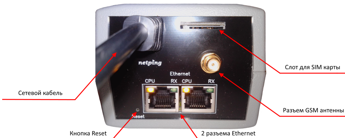
Рисунок 4 – Передняя панель (устройства NetPing 2/PWR-220 v1/SMS, NetPing 2/PWR-220 v2/SMS)
