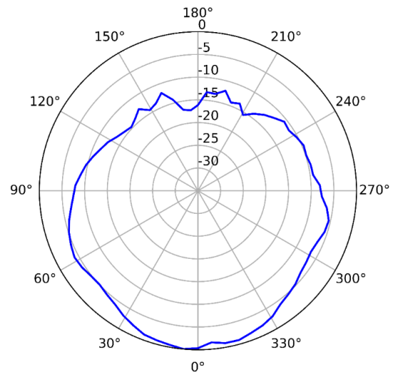
5GHz (Vertical)
