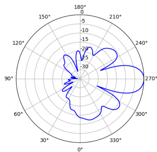
5GHz (Vertical)
