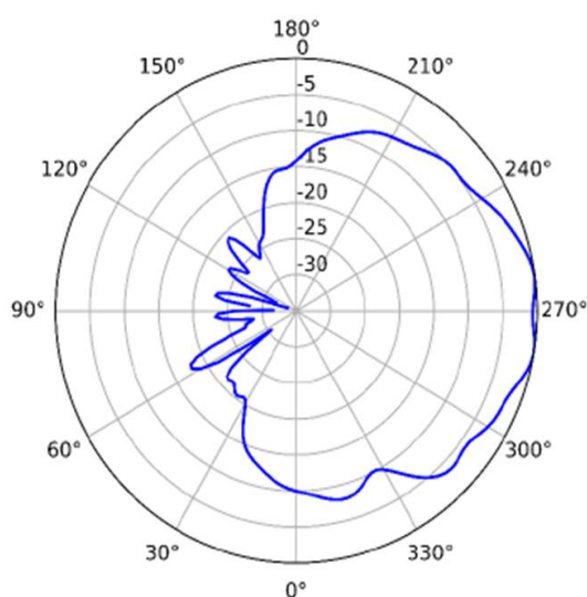
5GHz (Horizontal)
