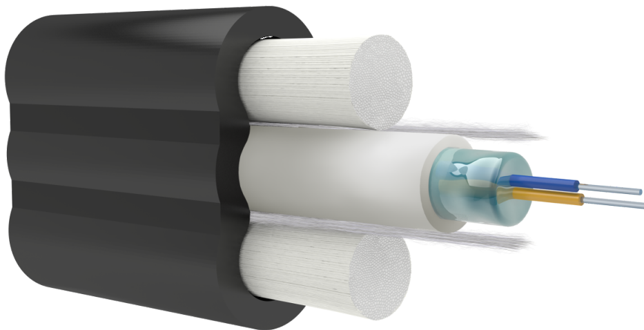
Рисунок 1 - Общий вид
