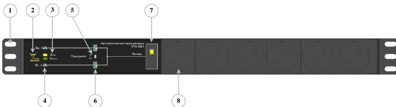
Рисунок 1 – Электронно-механический АВР ATS-1601(P), передняя панель:
