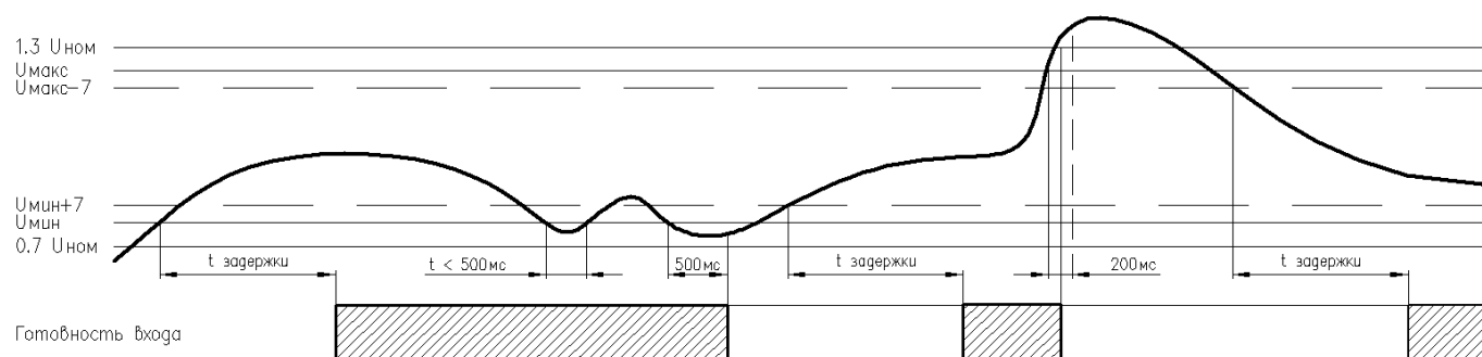
Рисунок 1 – Поясняющая диаграмма времени задержки и готовности входа.
