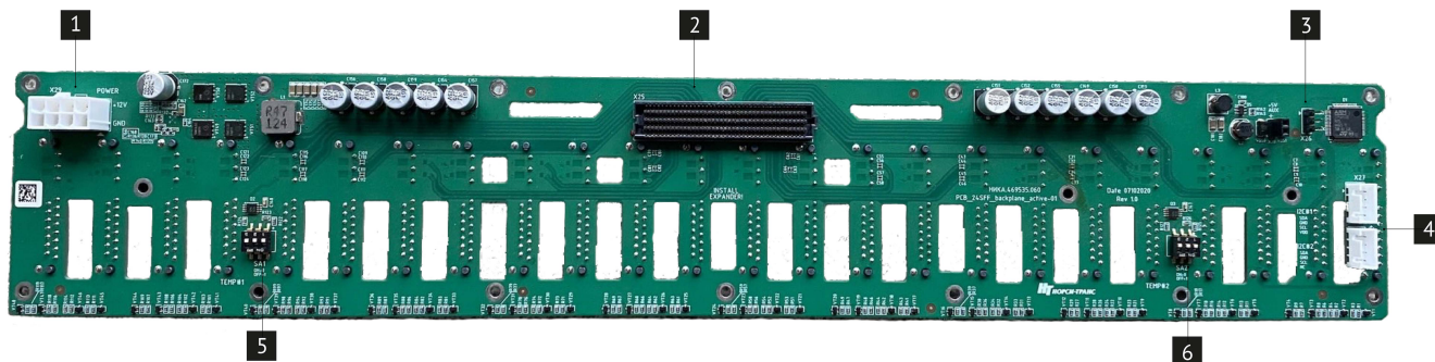
Рис. 14. Плата объединительная 24SFF (НИКА.469535.060)
