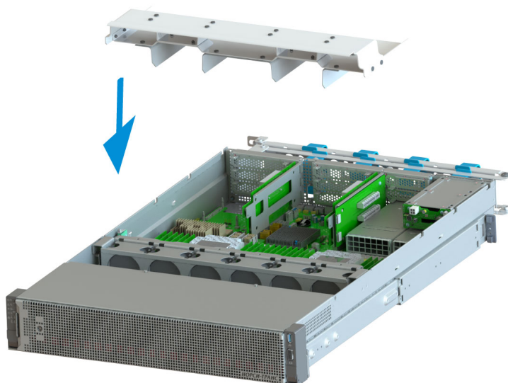
Рис. 25. Установка воздушного кожуха
