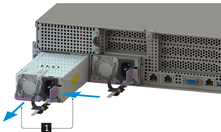
Рис. 54. Извлечение блока питания
