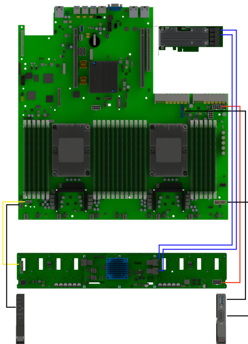
Рис. 29. Схема прокладки системных кабелей и кабелей питания с подключением PCIe RAID
