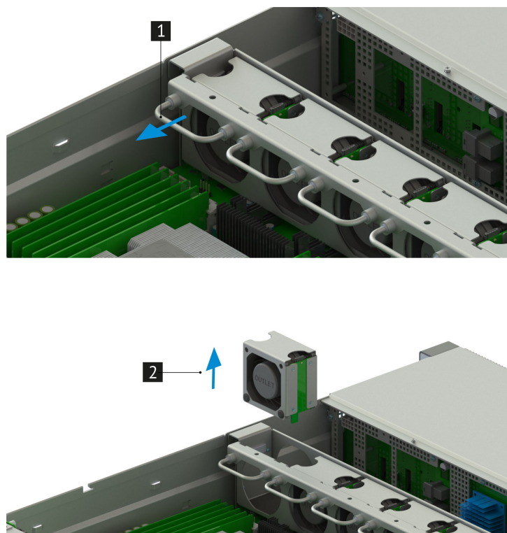
Рис. 31. Извлечение вентилятора
