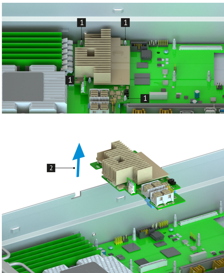
Рис. 45. Снятие наплатного RAID-контроллера
