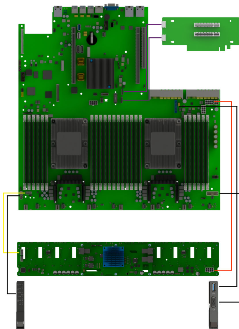
Рис. 30. Схема прокладки системных кабелей и кабелей OcuLink только в случае подключения Райзера 3x16-8-8 (НИКА.469535.047)
