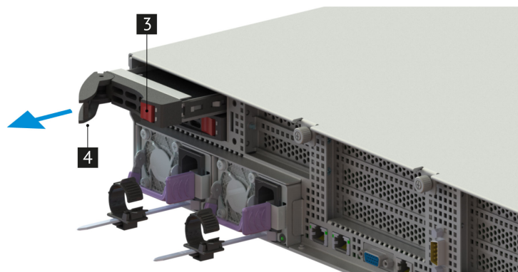
Рис. 44. Извлечение дисков
