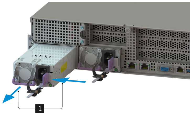
Рис. 52. Извлечение блока питания
