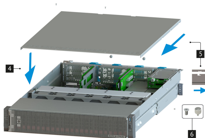
Рис. 23. Установка верхней крышки платформы
