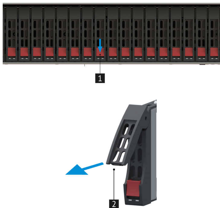
Рис. 42. Извлечение дисков
