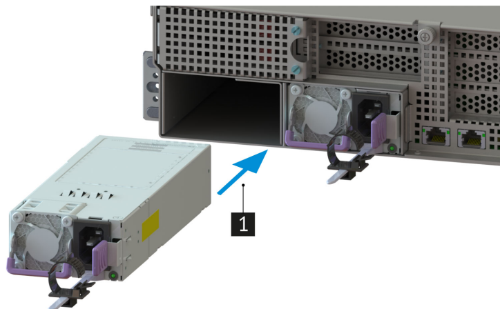
Рис. 53. Установка блока питания
