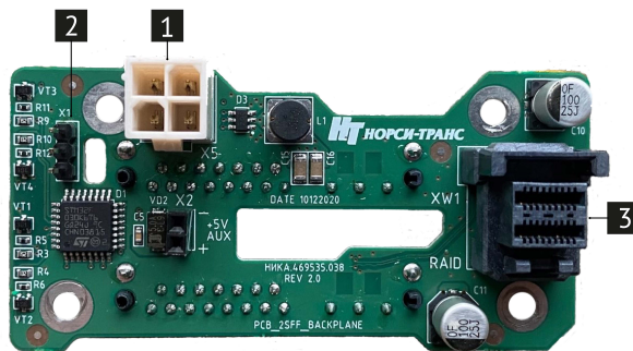
Рис. 15. Плата расширения 2SFF (НИКА.469535.038)
