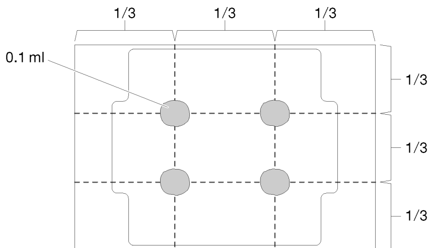
Рис. 39. Нанесение термопасты
