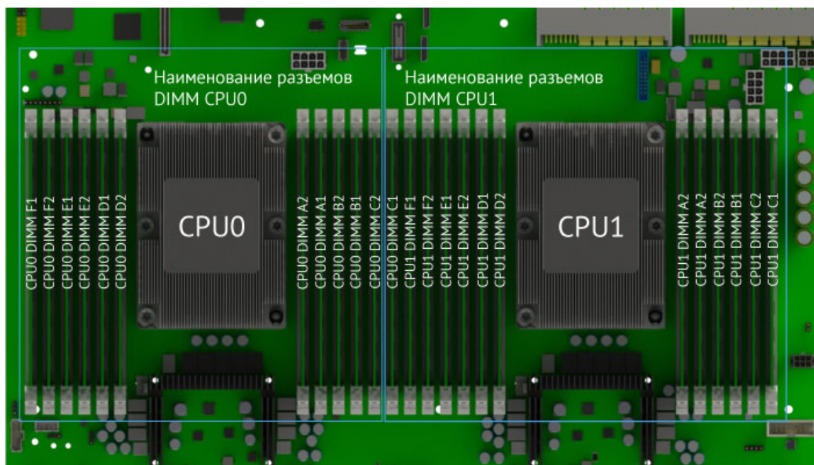
Рис. 33. Расположение разъемов
