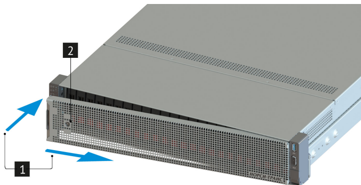
Рис. 21. Установка передней панели
