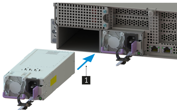
Рис. 55. Установка блока питания
