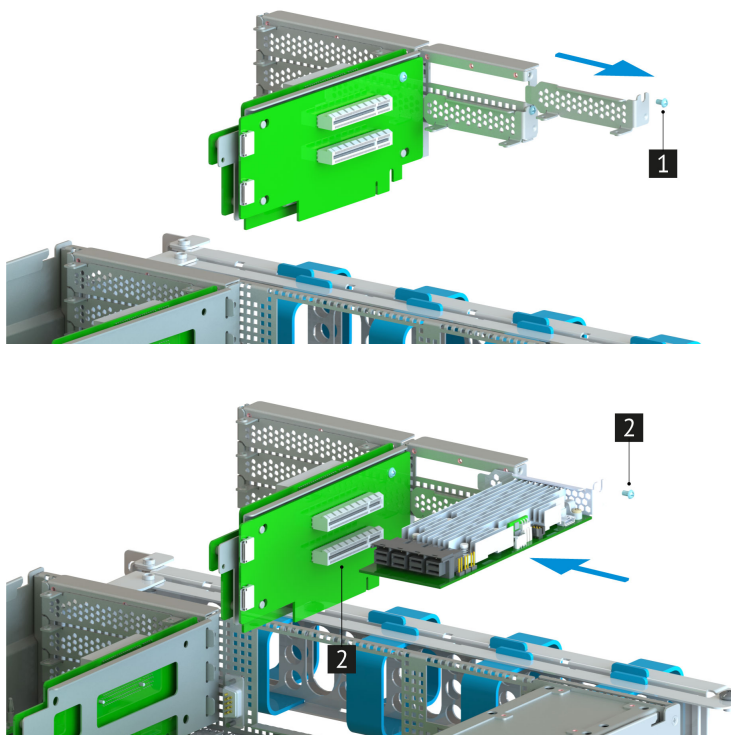
Рис. 47. Установка HBA/RAID-контроллера в PCIe-рейзере
