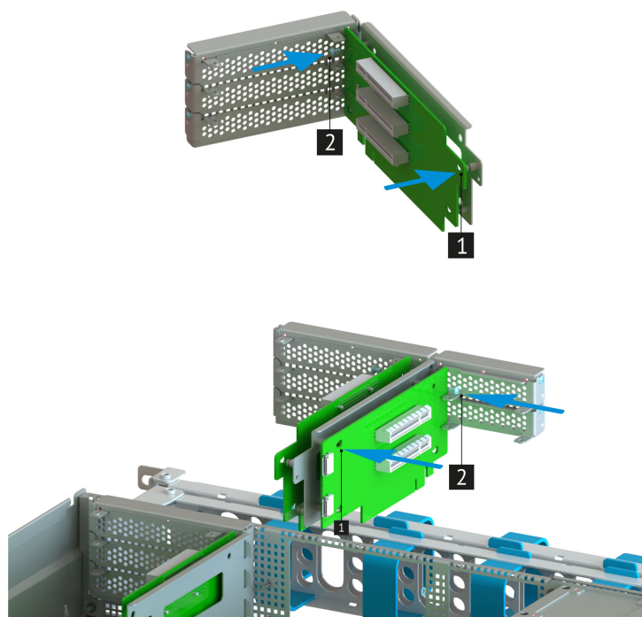
Рис. 48. Установка PCIe-райзера на основании
