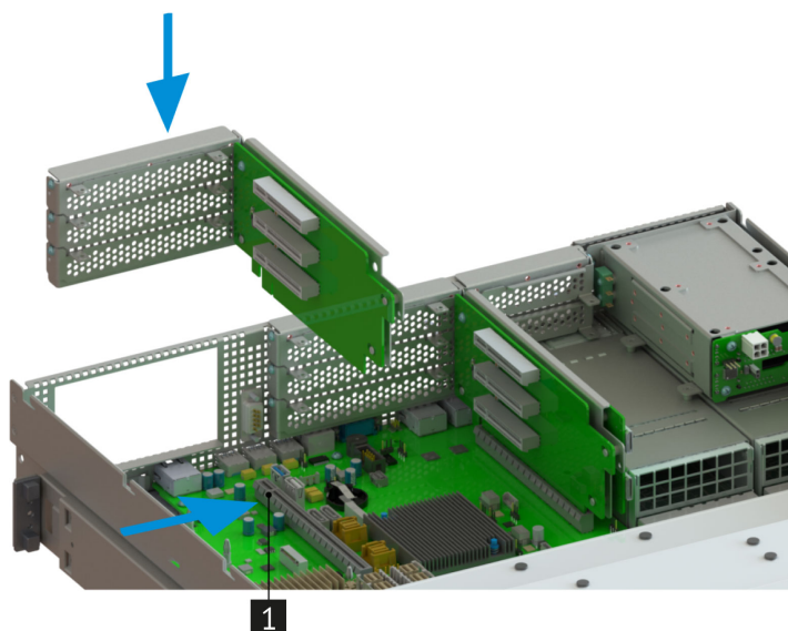
Рис. 49. Установка PCIe-райзера с основанием в корпус сервера
