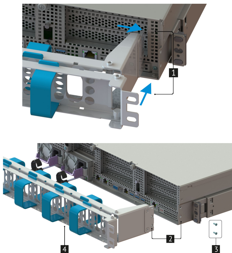
Рис. 19. Установка дополнительного кабельного органайзера.
