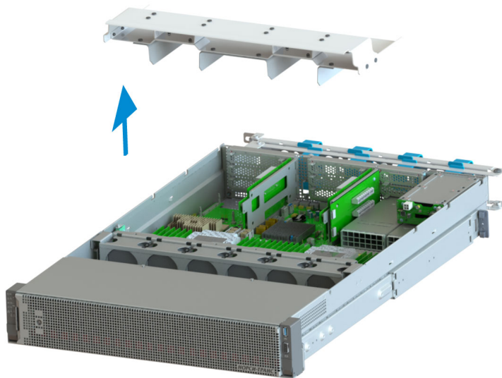
Рис. 24. Снятие воздушного кожуха
