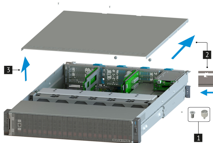
Рис. 22. Снятие верхней крышки платформы
