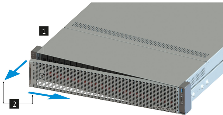
Рис. 20. Снятие передней панели
