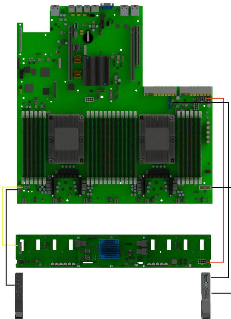
Рис. 27. Схема прокладки системных кабелей и кабелей питания
