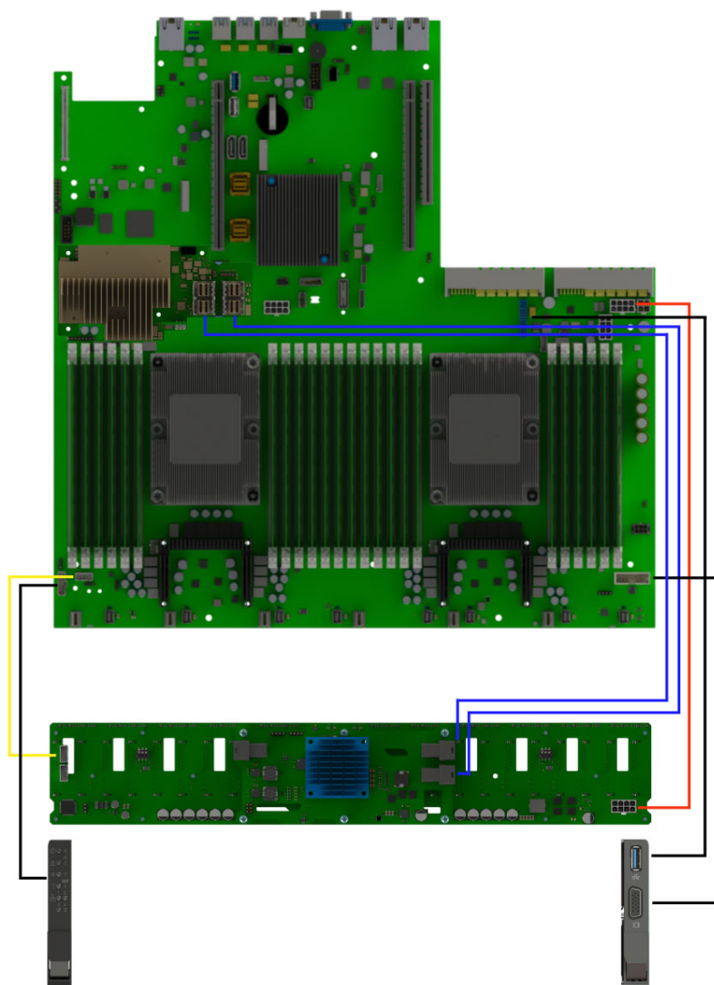
Рис. 28. Схема прокладки системных кабелей и кабелей питания с подключением наплатного RAID
