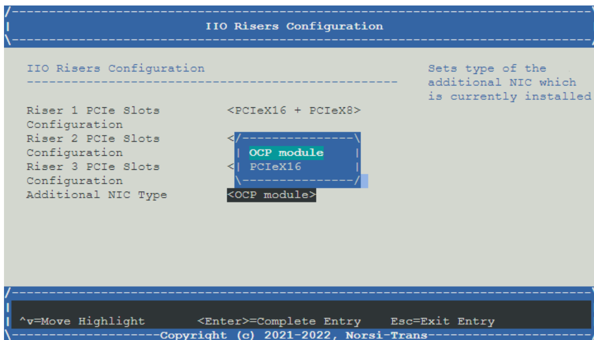
Рис. 67. Меню IIO Risers Configuration
