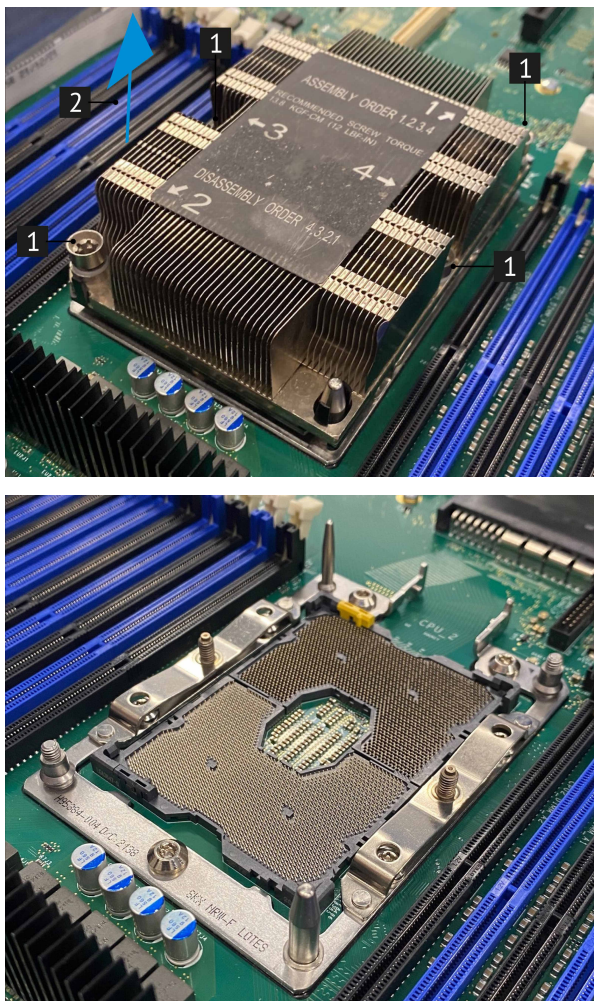
Рис. 36. Снятие модуля процессора с радиатором
