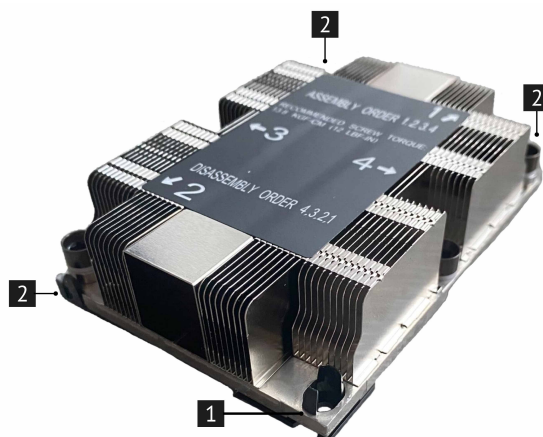
Рис. 37. Снятие процессора с радиатора
