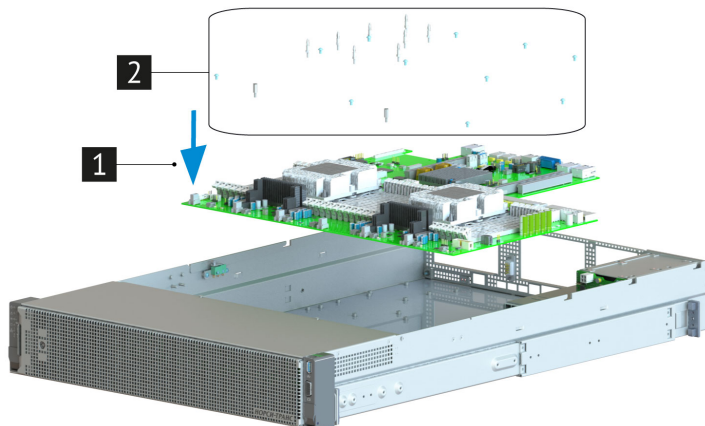
Рис. 41. Установка материнской платы
