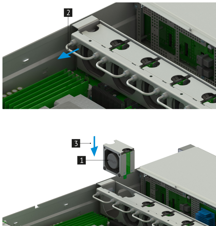
Рис. 32. Подключение вентилятора
