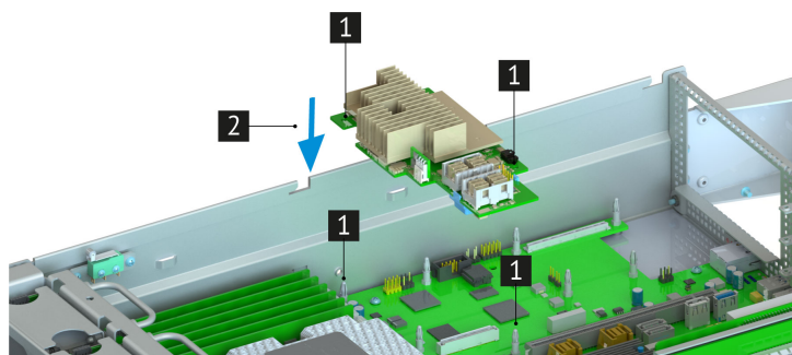
Рис. 46. Установка наплатного RAID-контроллера
