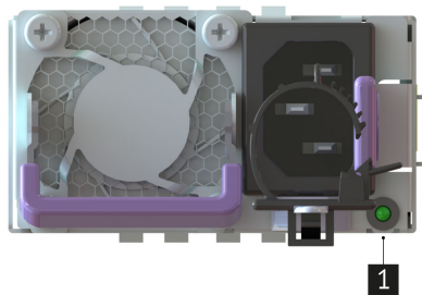
Рис. 51. Светодиодная индикация состояния блока питания
