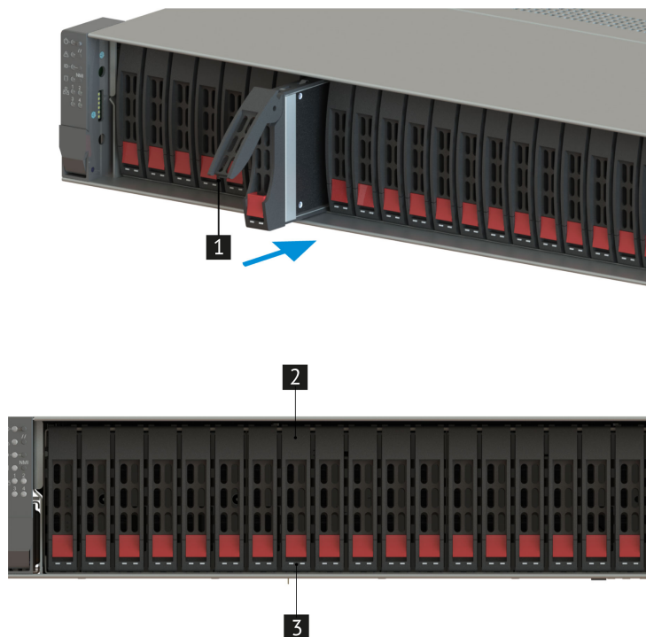
Рис. 43. Извлечение дисков
