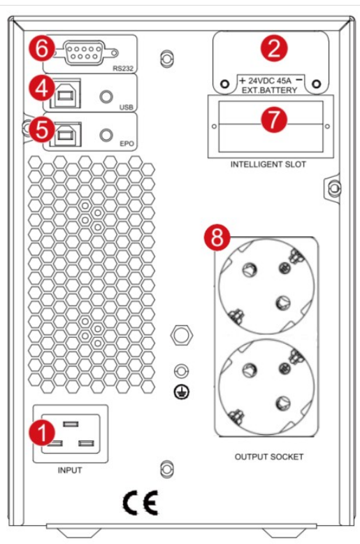
Рисунок 1 - SNR-UPS-ONT-1000-B36
