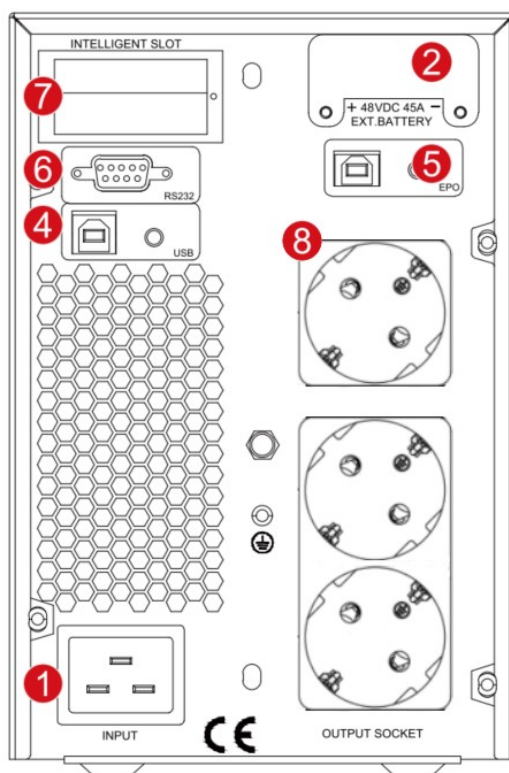
Рисунок 2 - SNR-UPS-ONT-2000-B48
