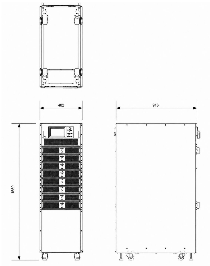
Рисунок 2 – Габаритные размеры
