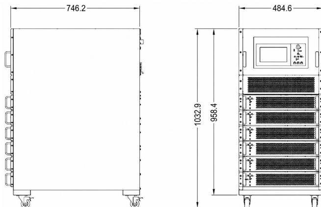
Рисунок 5 – Габаритные размеры
