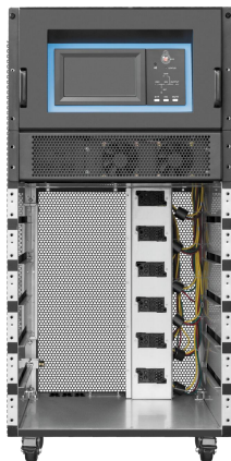
Рисунок 4 – ИБП без силовых модулей
