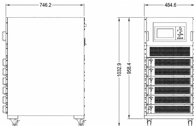
Рисунок 5 – Габаритные размеры
