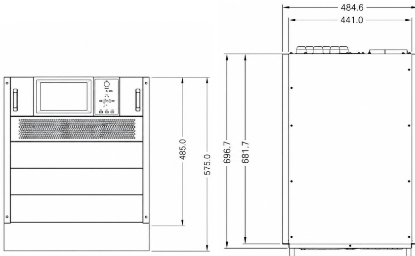
Рисунок 5 – Габаритные размеры
