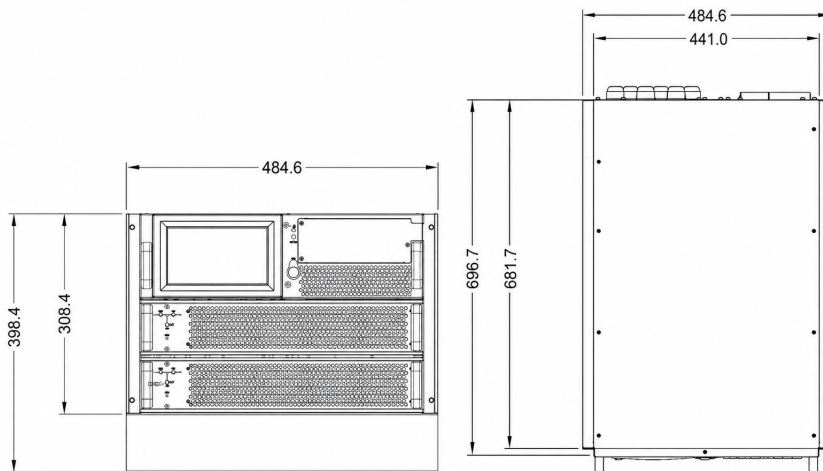
Рисунок 2 – Габаритные размеры
