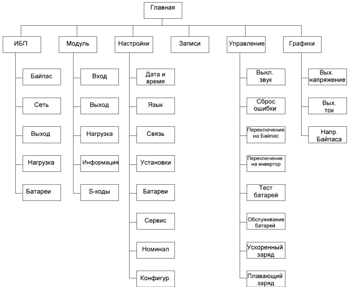
Рис. 7-3: Структура меню
