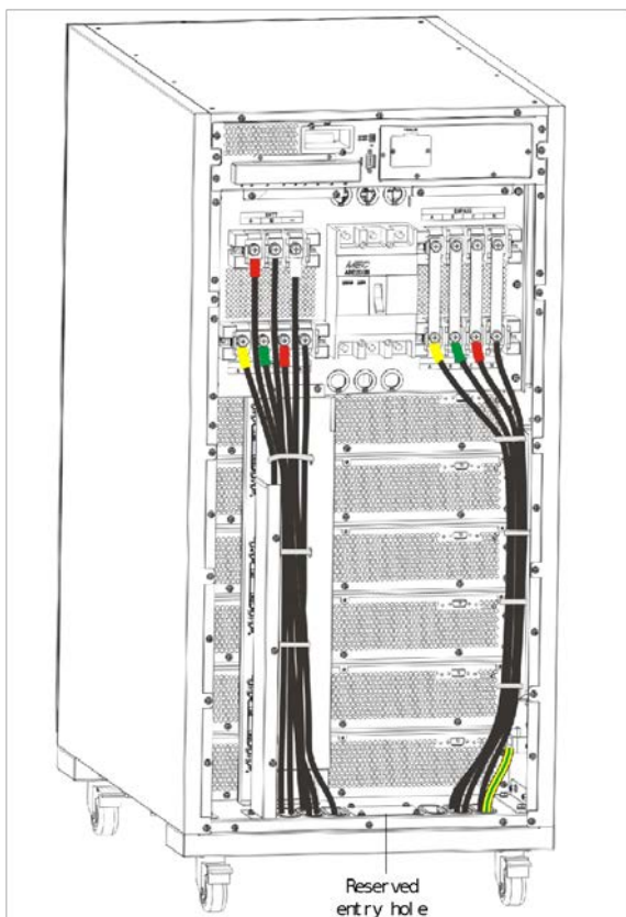
(а) Кабельный ввод в 6 модульном шасси Рисунок 7 – Кабельные вводы
