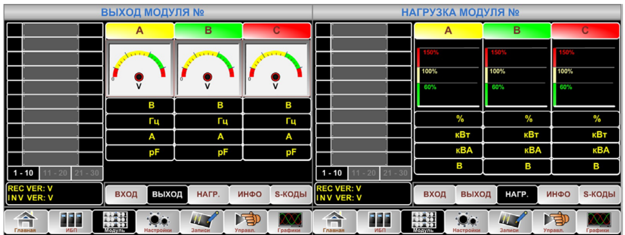
(а) информация о выходе модуля (б) информация о загрузке модуля
