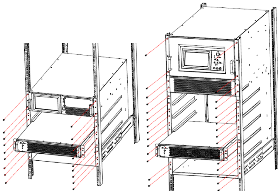
(б) Установка ИБП в серверный шкаф Рисунок 6 – Установка ИБП в серверный шкаф
