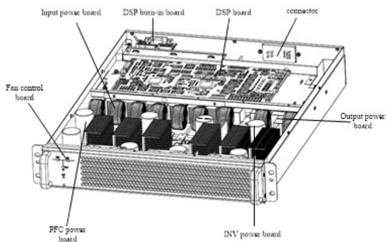
Рисунок 27 Модуль Байпаса
