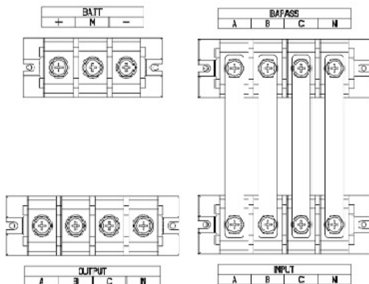
Схема подключения питания 60KVA/90KVA (б)
