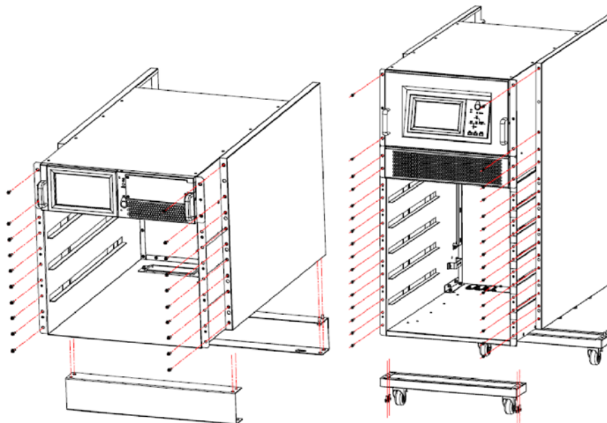
(a) Снятие боковых панелей и консоли
