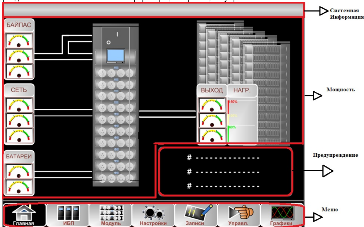
Рис. 7-2 ЖК-дисплей
