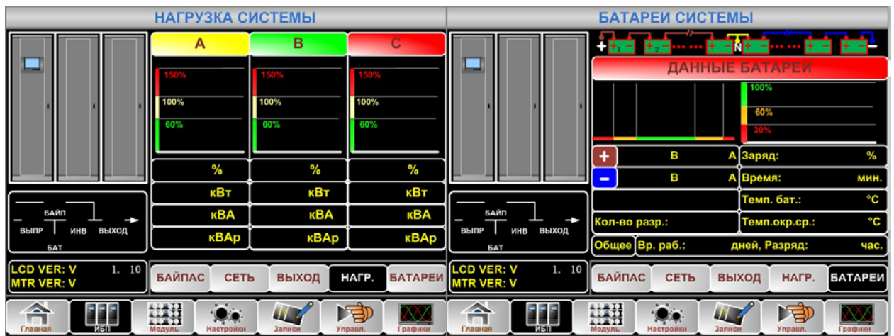
(а) информация о загрузке системы (б) информация об аккумуляторах Рис.7-6: информация о нагрузке и батарее
