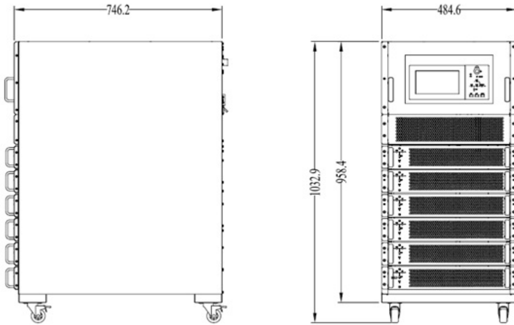
Рисунок 24 Внешние размеры ИБП
