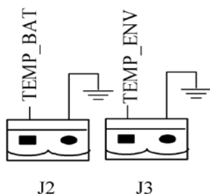
Рисунок 10 – Схема сухих контактов J2 и J3, предназначенных для контроля температуры Таблица 1-3. Описание входных интерфейсов с сухими контактами J2 и J3
