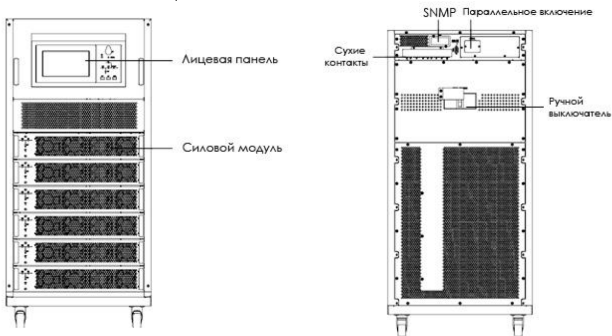
Рисунок 1 – Шасси ИБП с 6 силовыми модулями
