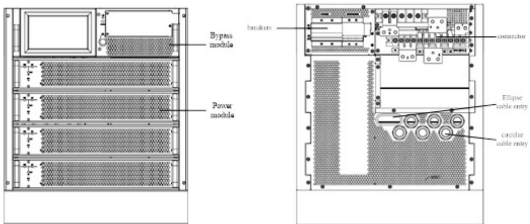
Рисунок 23 Модули ИБП вид спереди вид сзади
