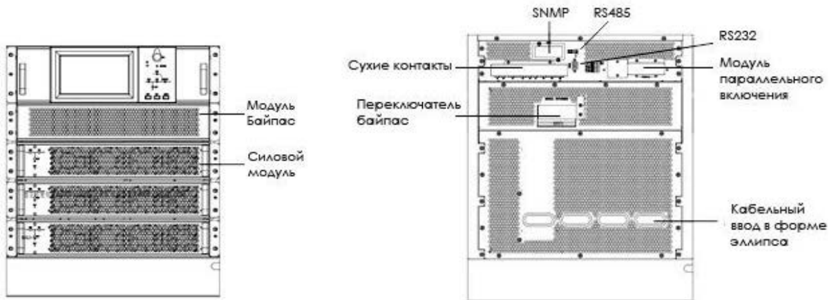
Рисунок 3 – Шасси ИБП с 3 силовыми модулями
