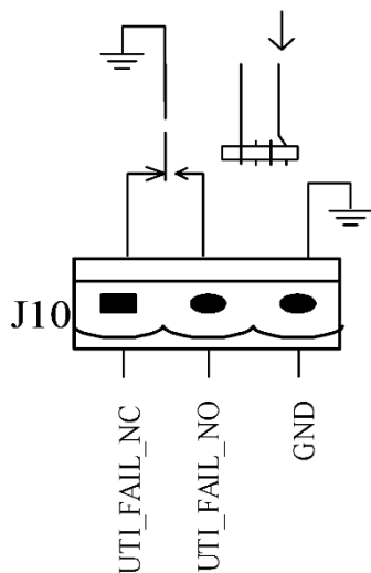
Рисунок 16 - Схема интерфейса с сухими контактами для предупреждения о неисправности сети Таблица 1-9. Описание интерфейса с сухими контактами для предупреждения о неисправности сети
