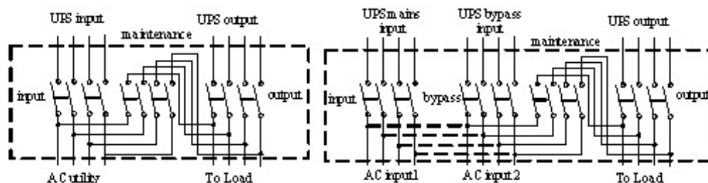
(a) Единый вход (b) Вход для разделения байпаса рисунок 31 Внешний Bypass.
