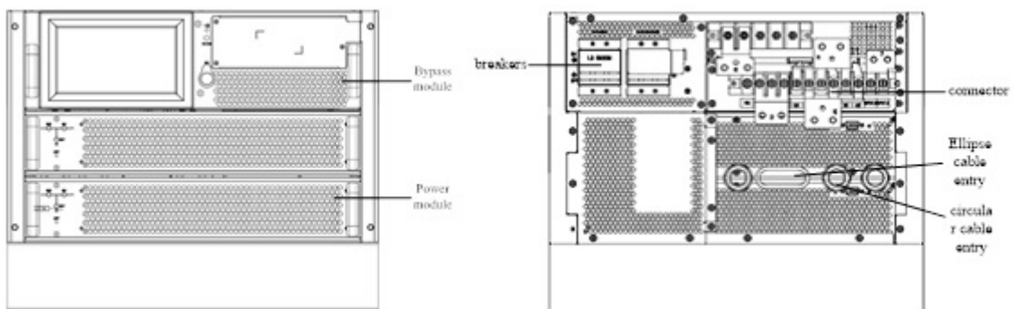
Рисунок 23 Модули ИБП вид спереди вид сзади
