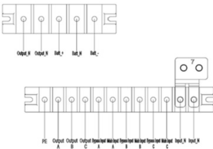
Схема подключения питания 20KVA/40KVA (a)
