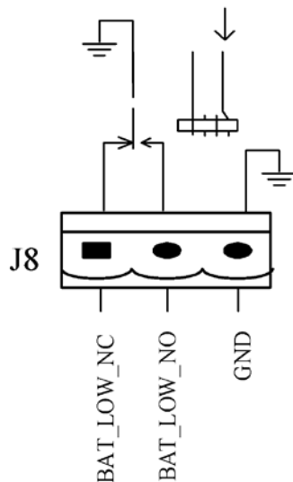
Рисунок 14 – Схема интерфейса с сухими контактами для предупреждения о состоянии аккумулятора Таблица 1-7. Описание интерфейса с сухими контактами для предупреждения о состоянии аккумулятора
