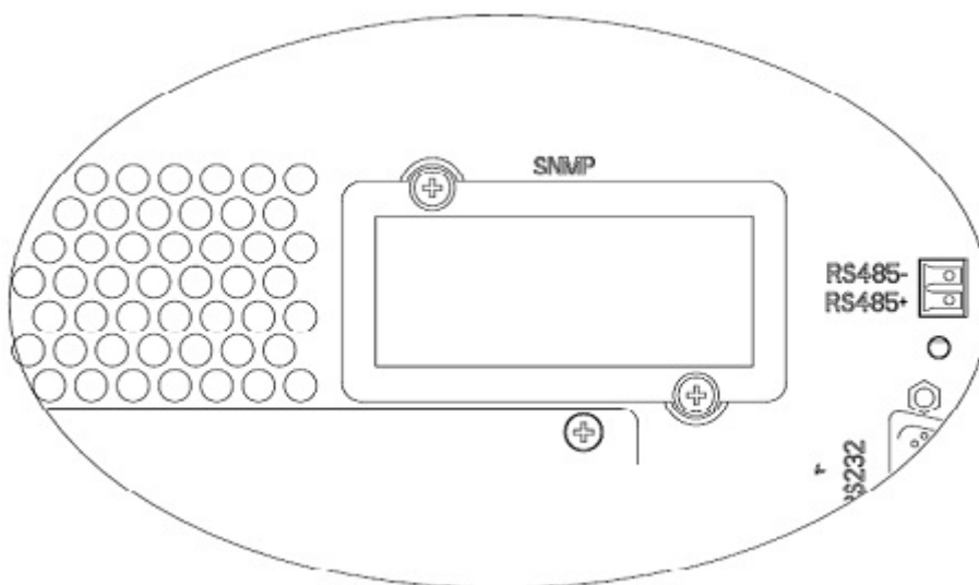
Рис.8-1: Установка SNMP-карта
