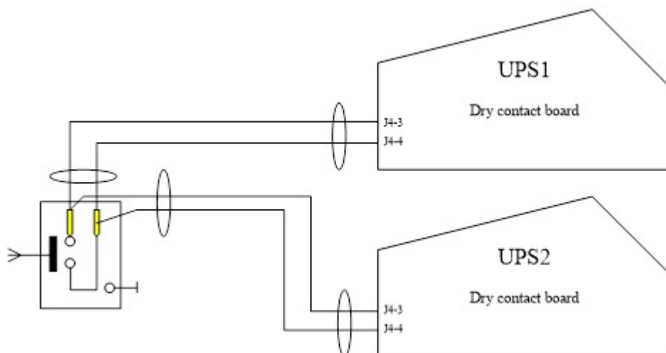
2) Параллельное подключение
