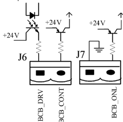
Рисунок 13 - Интерфейс BCB
