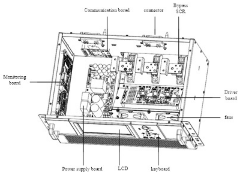
б) Модуль Байпаса 30KVA/45KVA
