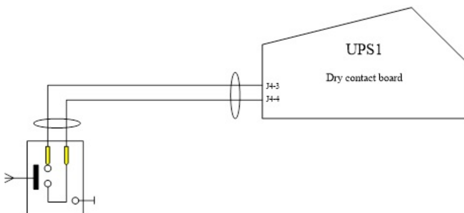
Единичное подключение
