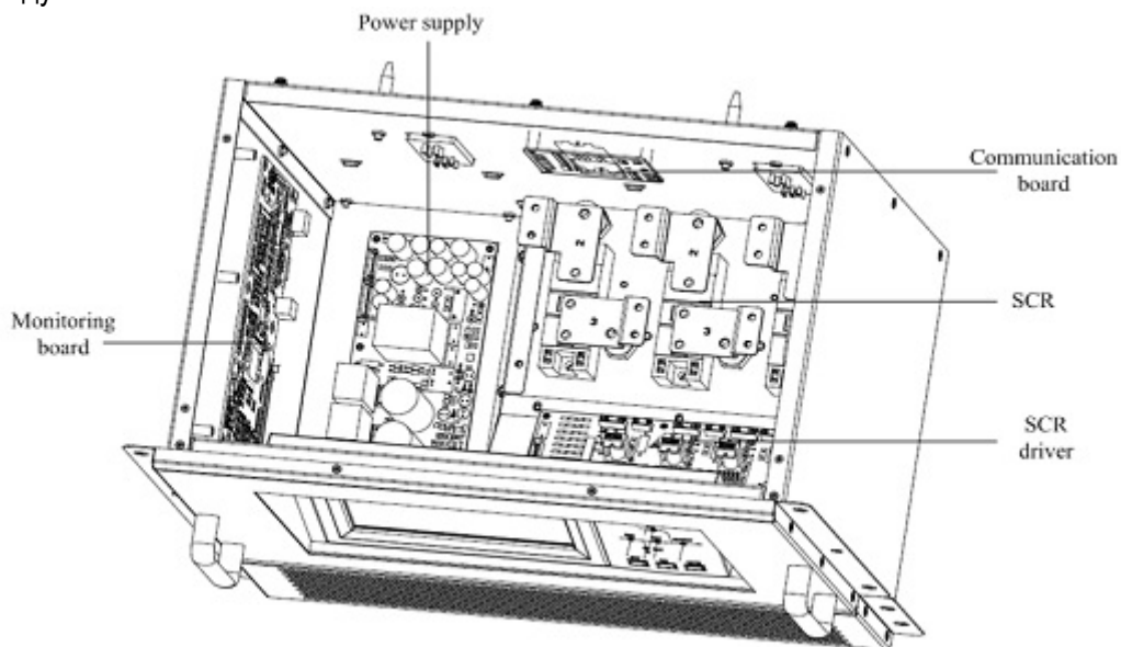
с) Модуль Байпаса 60KVA/90KVA
