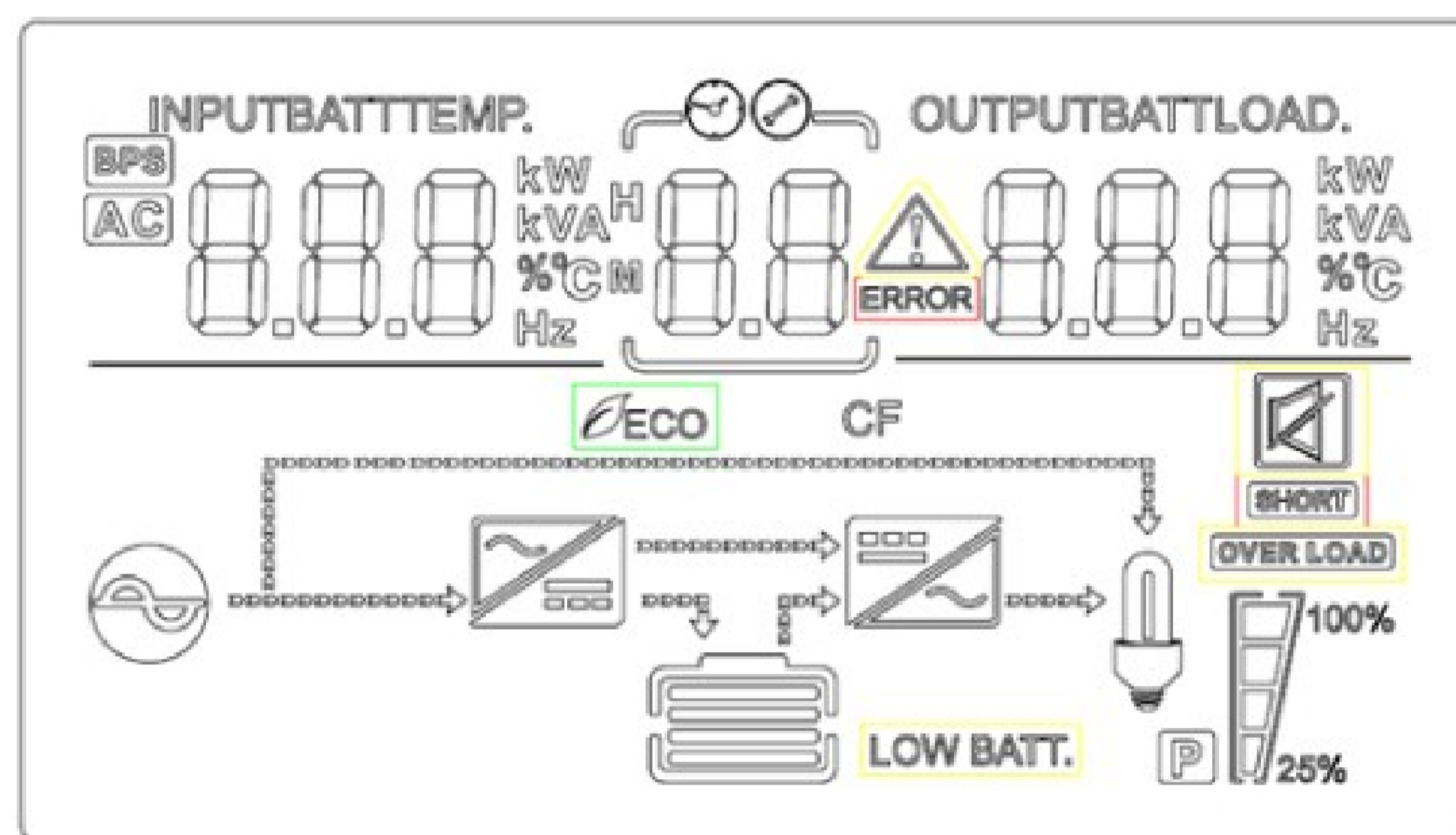
Рис. 18 — ЖК-дисплей
