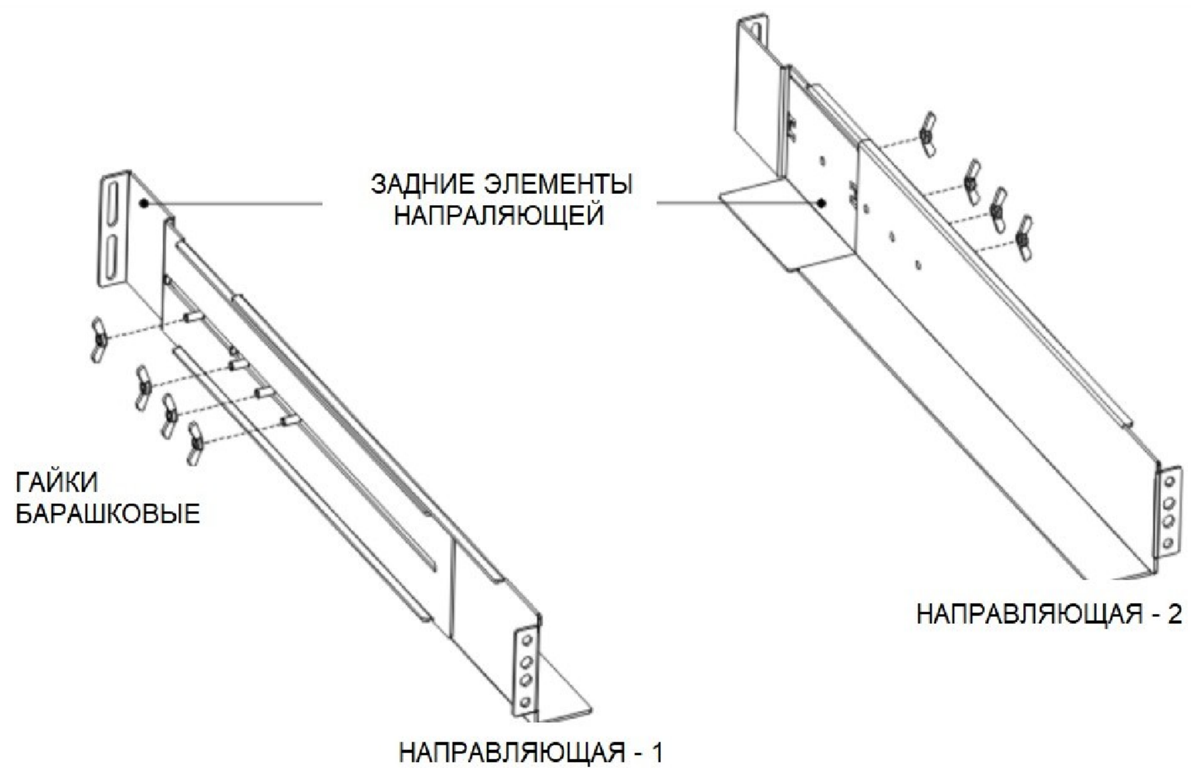
Рис.5 — Сборка направляющих
