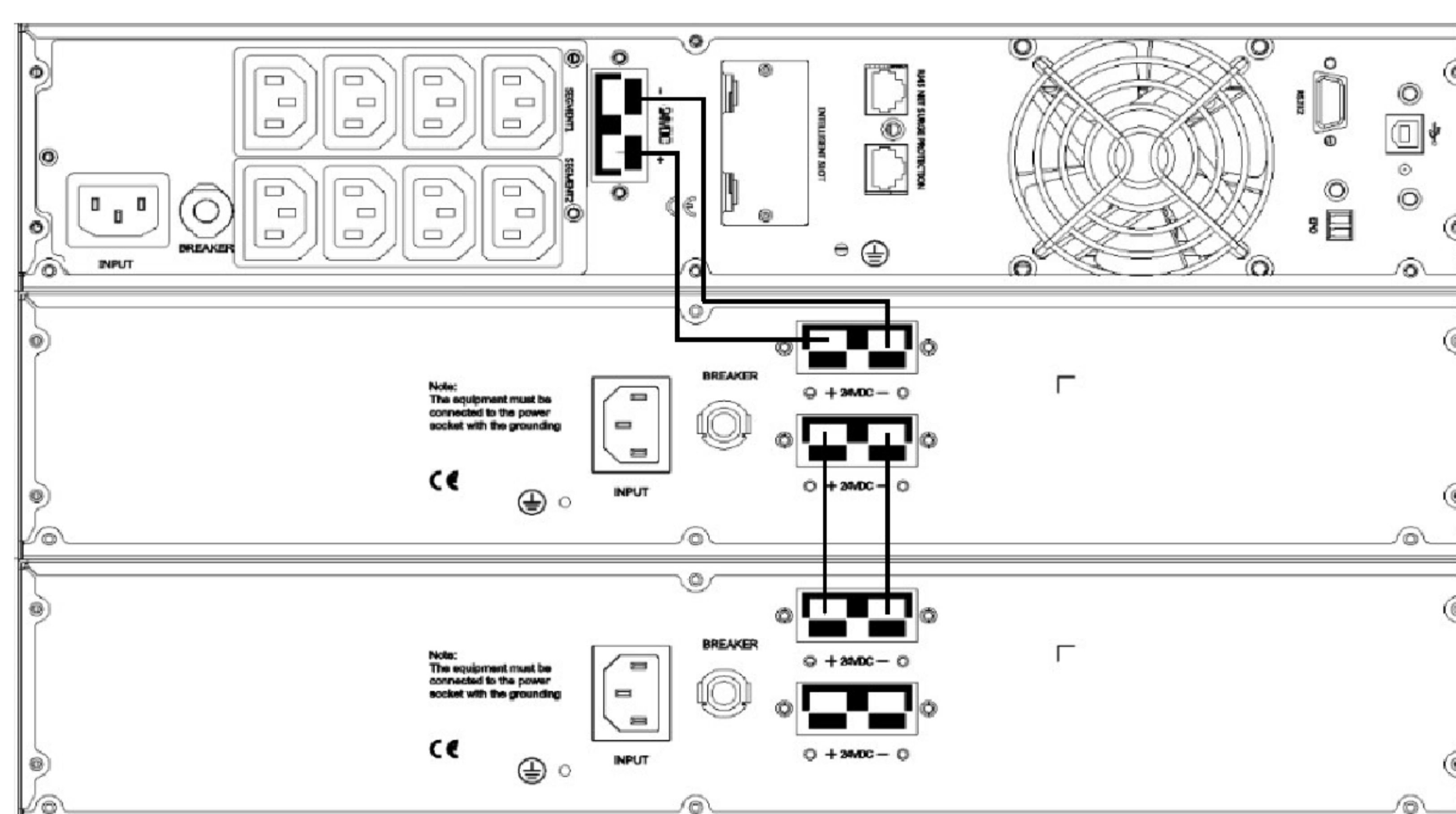
Рис.14 — Схема подключения дополнительных блоков батарей
