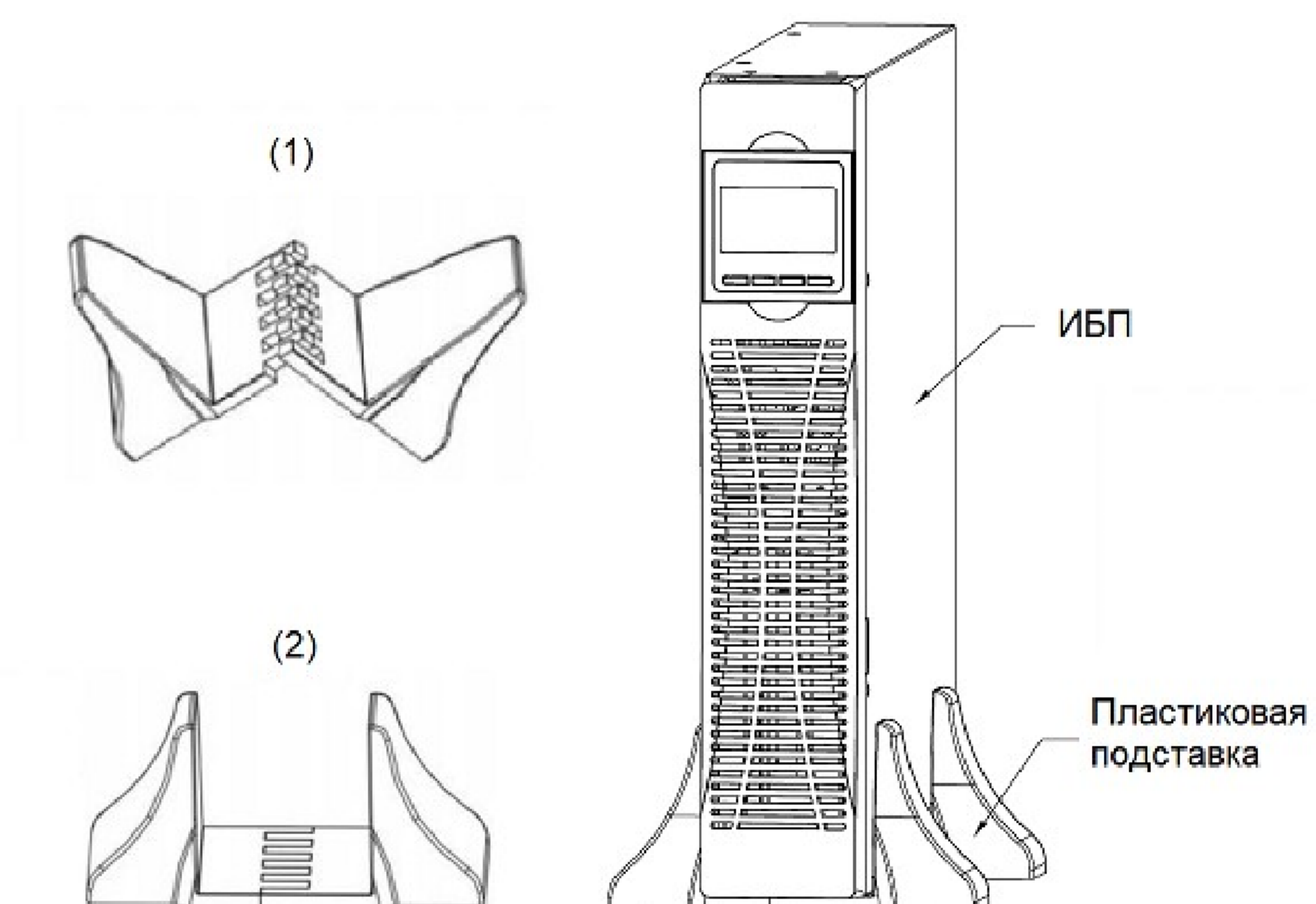
Рис.9 - Сборка подставок для установки ИБП в вертикальном положении
