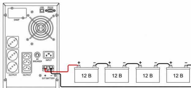
Рисунок 4 – Подключение цепи АКБ к ИБП
