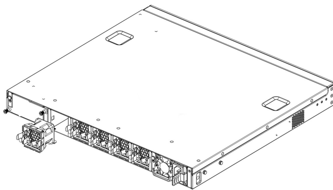
Рисунок 3.3 - Установка блока вентилятора охлаждения
