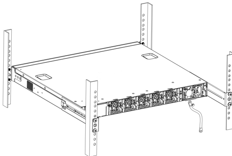
Рисунок 3.7 - Подключение кабеля заземления.
