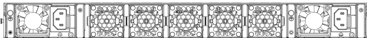
Рисунок 1.4- Задняя панель коммутатора SNR-S4550-24XQ в полной комплектации.
