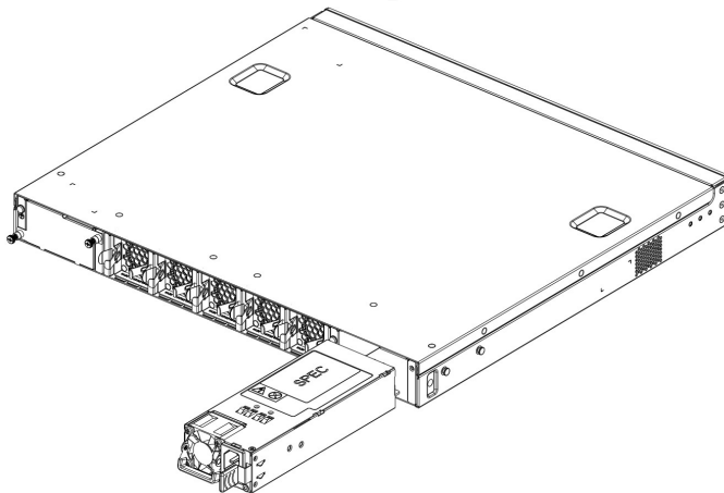
Рисунок 3.2 - Установка блока питания
