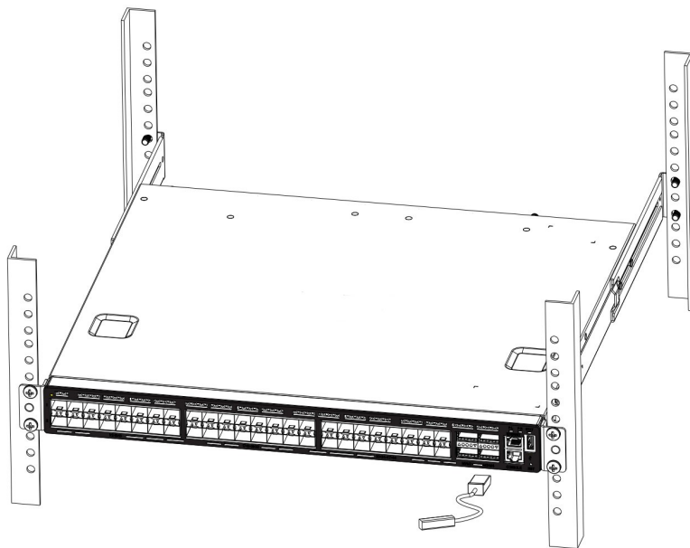
Рисунок 3.5 - Подключение кабеля DAC
