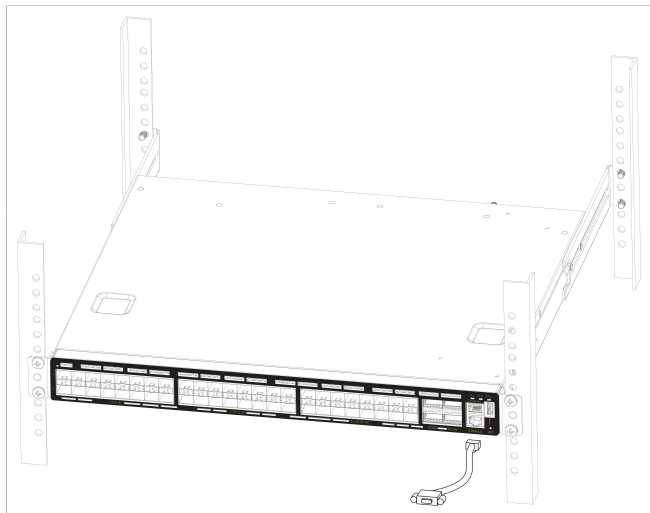
Рисунок 3.4 - Подключение консольного кабеля к коммутатору SNR-S4550-24XQ
