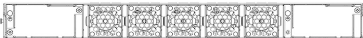
Рисунок 1.3 - Задняя панель коммутатора SNR-S4550-24XQ в стандартной комплектации.
