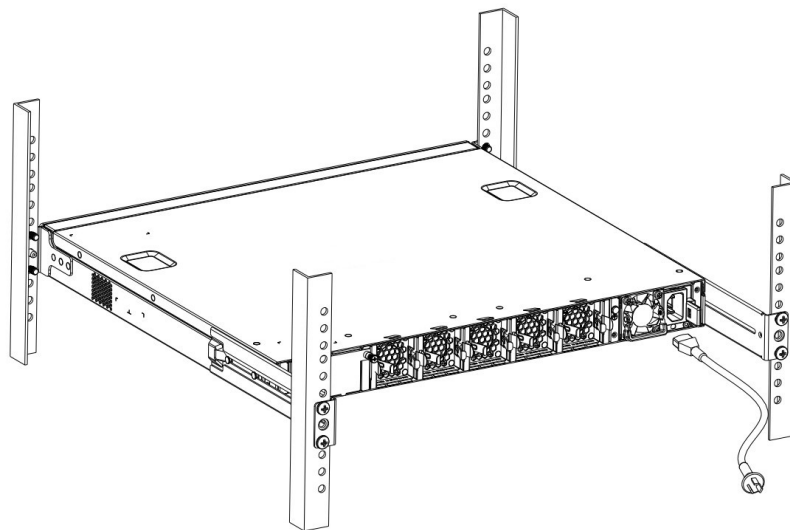
Рисунок 3.6 - Подключение кабеля электропитания.
