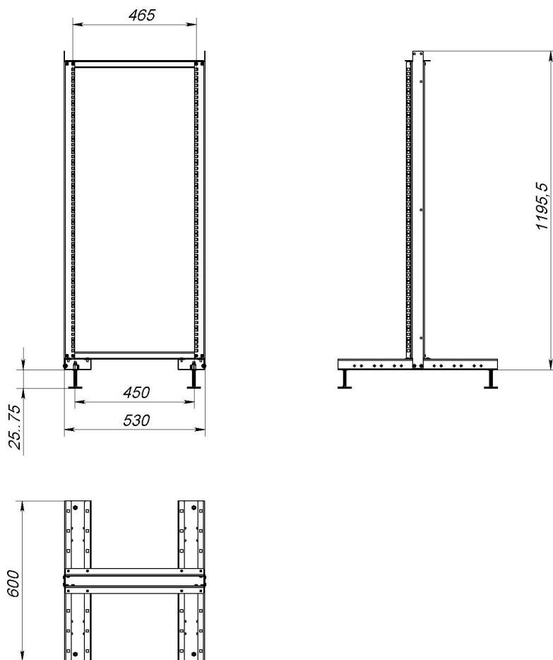
Рисунок 7– Чертеж. SNR-STK-0-6024
