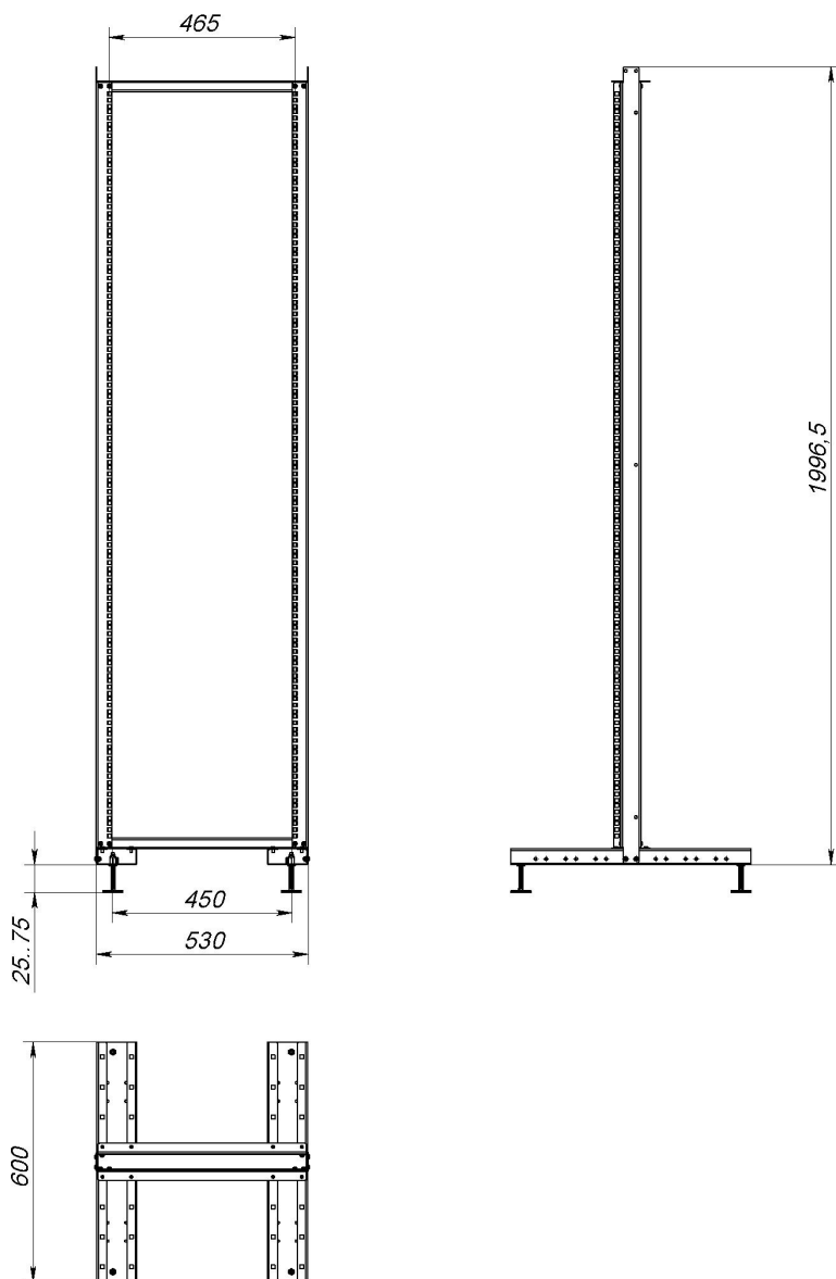
Рисунок 5 – Чертеж. SNR-STK-O-6042
