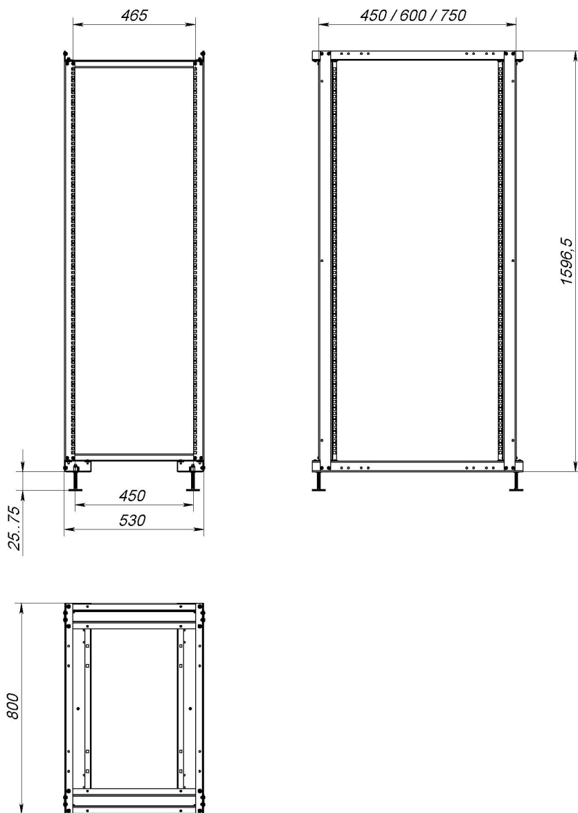
Рисунок 3 – Чертеж. SNR-STK-S-7533
