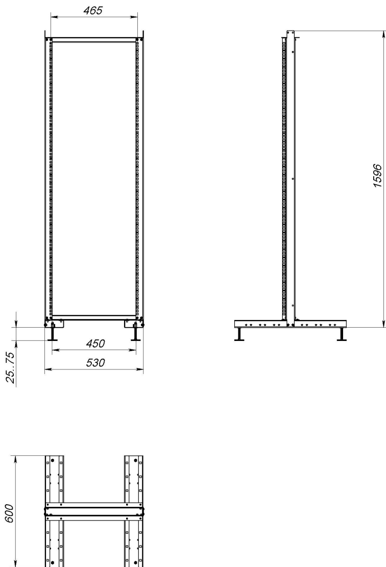
Рисунок 6 – Чертеж. SNR-STK-O-6033
