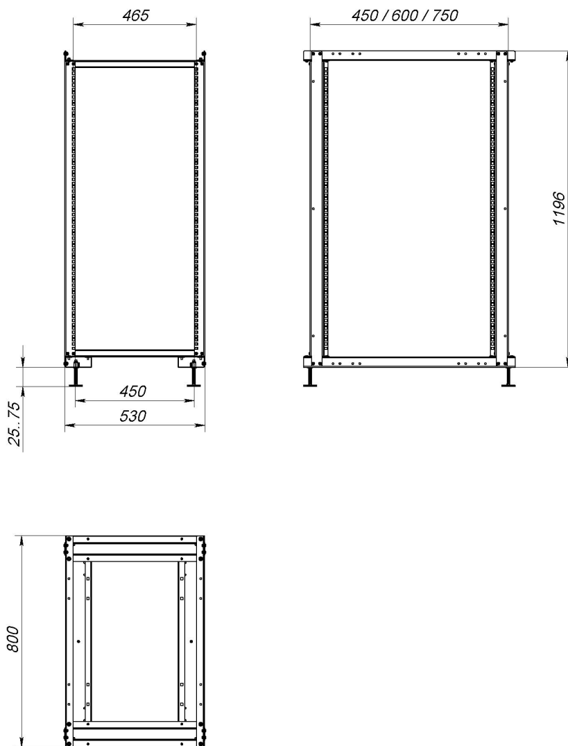
Рисунок 4 – Чертеж. SNR-STK-S-7524
