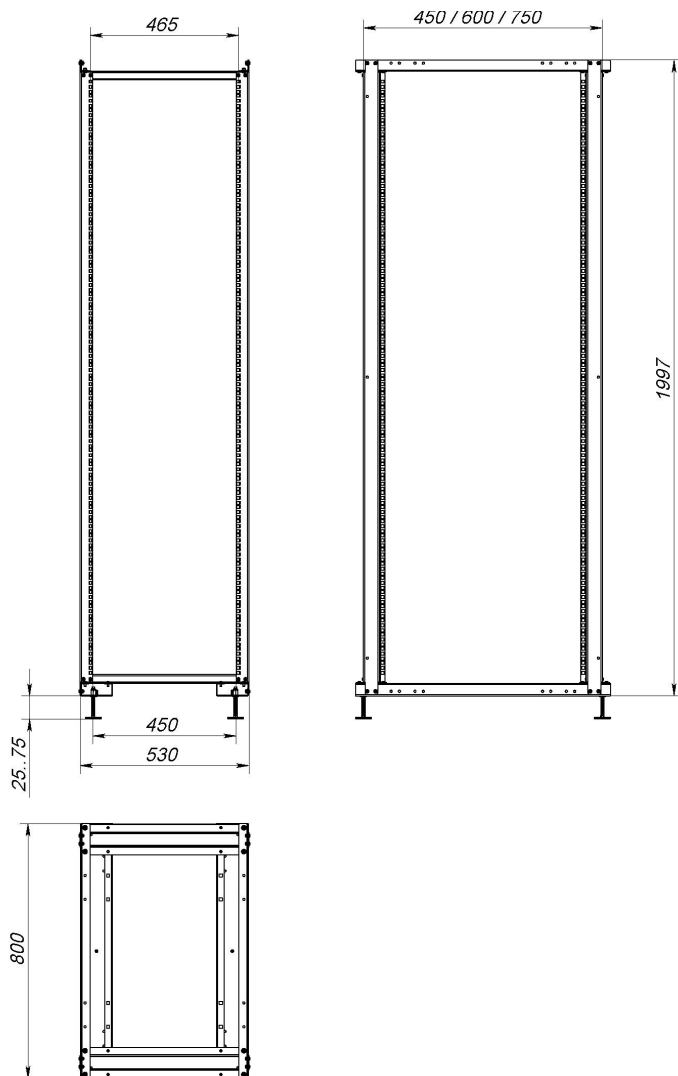
Рисунок 2 – Чертеж. SNR-STK-S-7542
