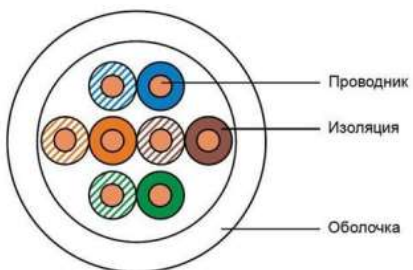
Рисунок 2 – Конструкция кабеля
