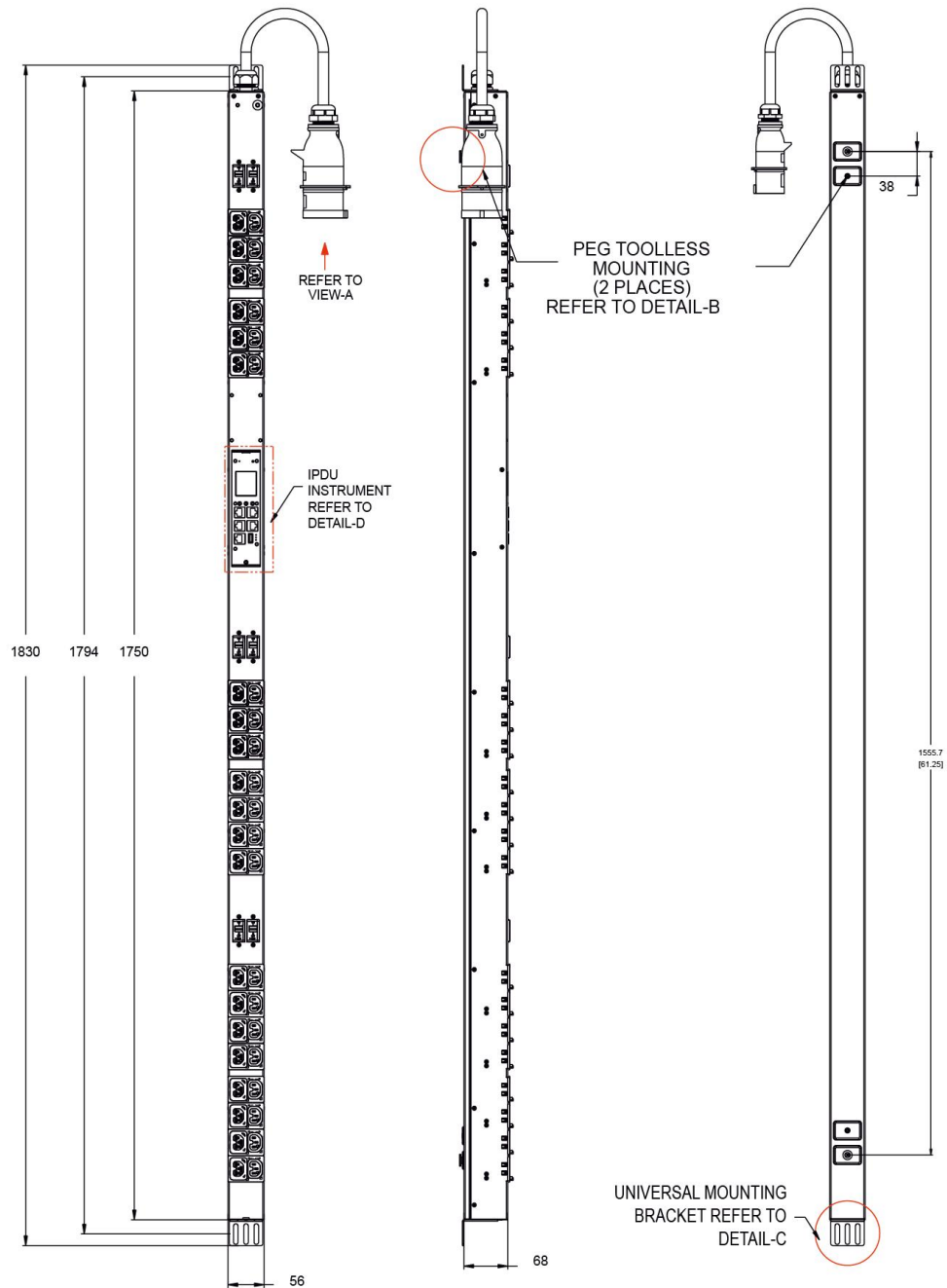
РИСУНОК 1 – ЧЕРТЕЖ УСТРОЙСТВА
