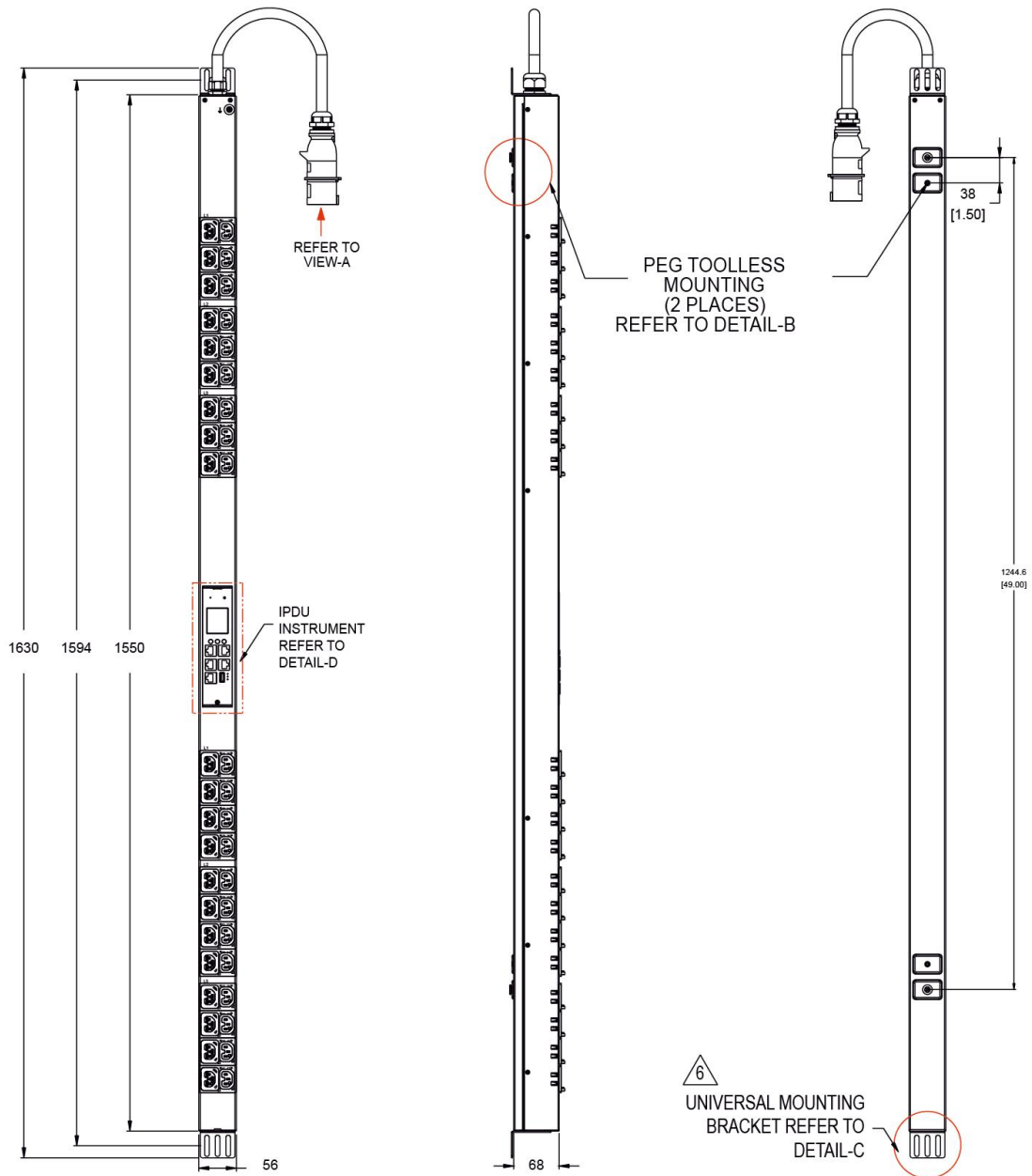
РИСУНОК 1 – ЧЕРТЕЖ УСТРОЙСТВА
