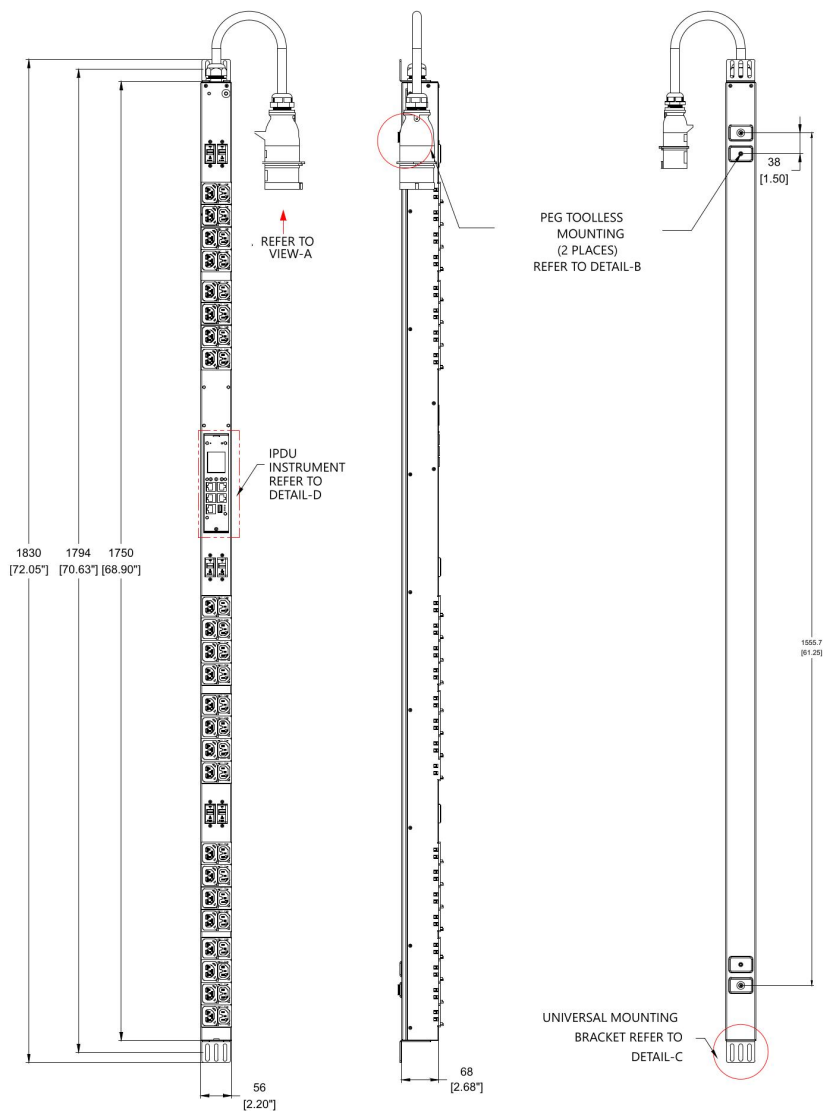
Рисунок 1 – Чертеж устройства
