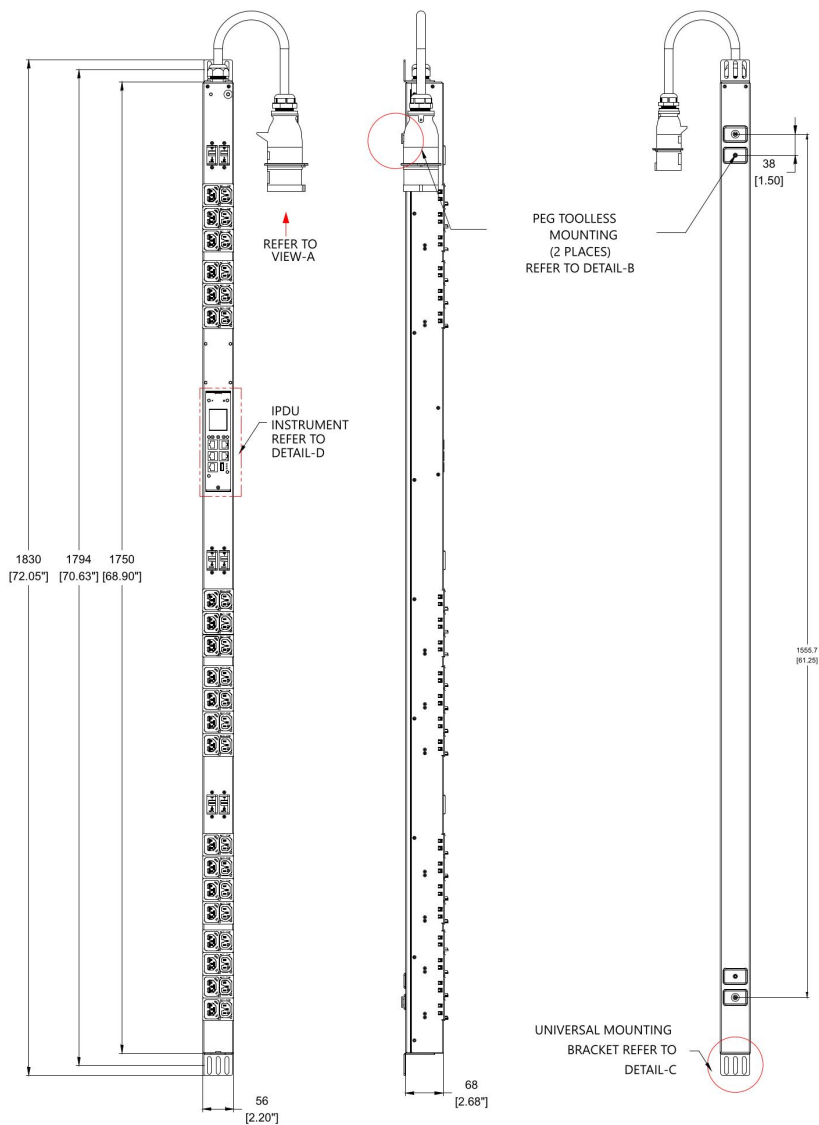
Рисунок 1 – Чертеж устройства
