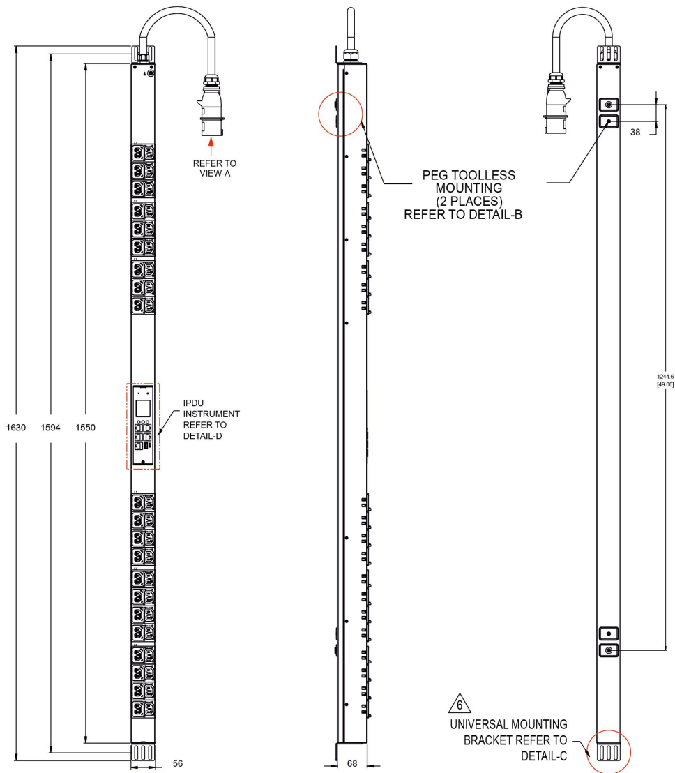
Рисунок 1 – Чертеж устройства
