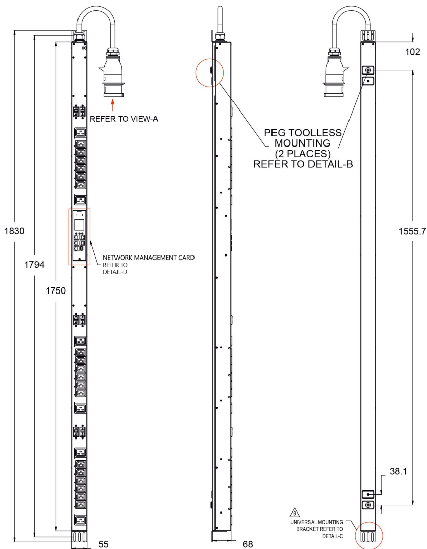
Рисунок 1 – Чертеж устройства
